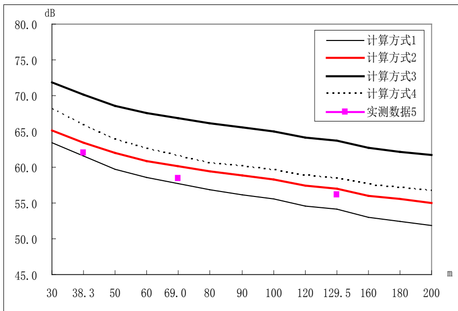
附图 1、交通噪声按不同预测模型计算与实测结果比较 (昼间) (2010 年)
