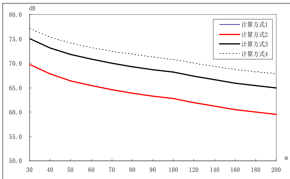
附图 1、交通噪声按不同计算方式昼间结果比较
