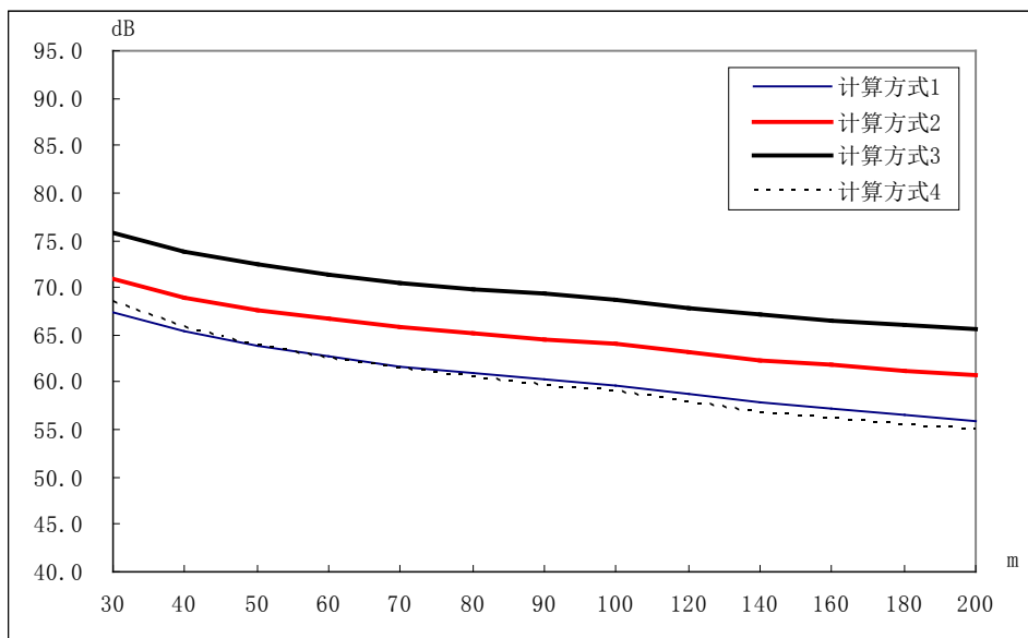
附图 1、交通噪声按不同计算方式昼间结果比较 (2012 年)
