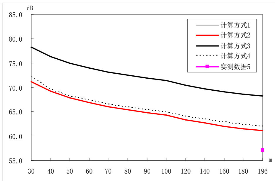
附图 1、交通噪声按不同计算方式昼间结果比较 (2010 年)
