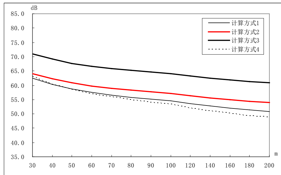
附图 2、交通噪声按不同计算方式夜间结果比较 (2012 年)
