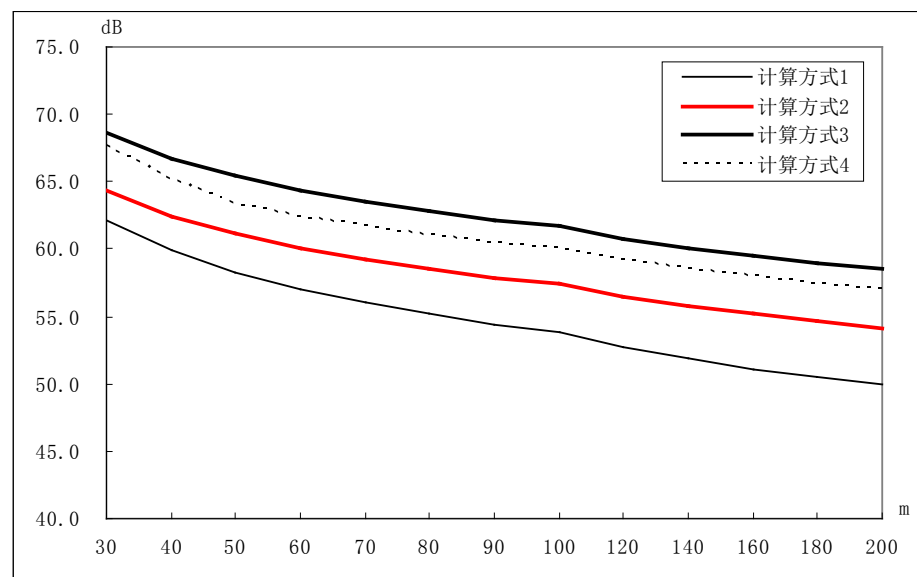
附图 2、交通噪声按不同计算方式夜间结果比较 (2011 年)
