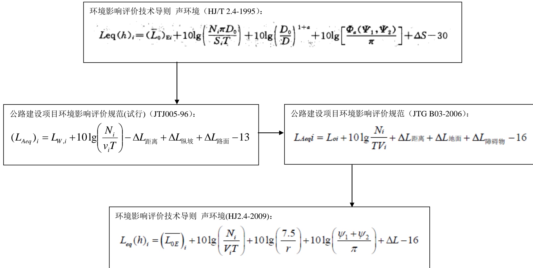
图 1 公路交通运输噪声预测基本模式的演变
