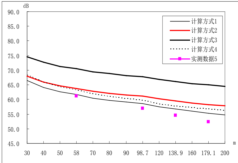
附图 1、交通噪声按不同计算方式结果比较（昼间） (2010 年)
