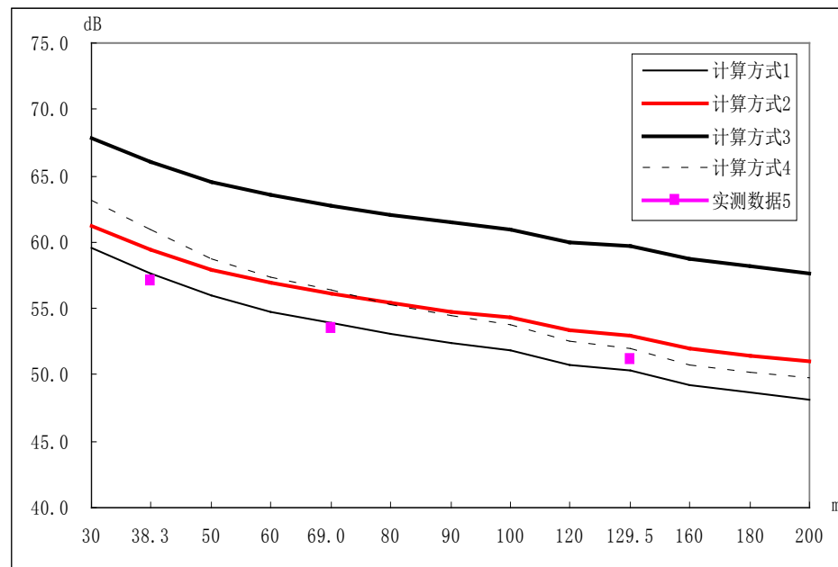
附图 2、交通噪声按不同预测模型计算与实测结果比较 (夜间) (2010 年)
