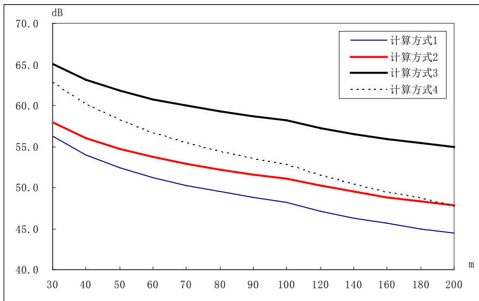
附图 1、交通噪声按不同计算方式日间结果比较 (2011 年)
