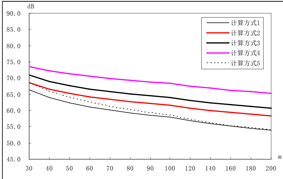
附图 1、交通噪声按不同计算方式昼间结果比较 (2014 年)
