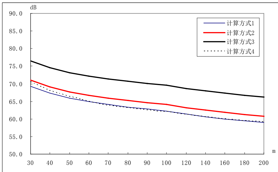
附图 1、交通噪声按不同计算方式昼间结果比较 (2011 年)
