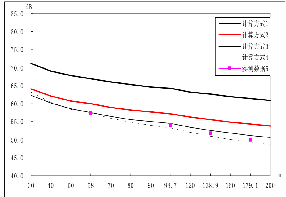
附图 2、交通噪声按不同计算方式结果比较（夜间） (2010 年)
