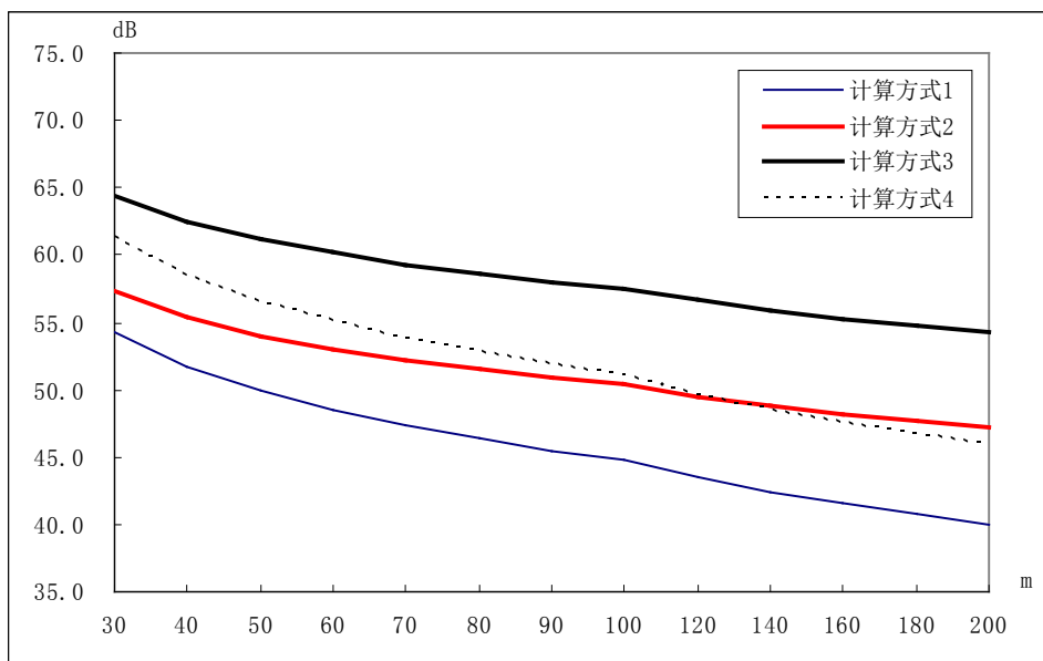
附图 1、交通噪声按不同计算方式昼间结果比较 (2012 年)
