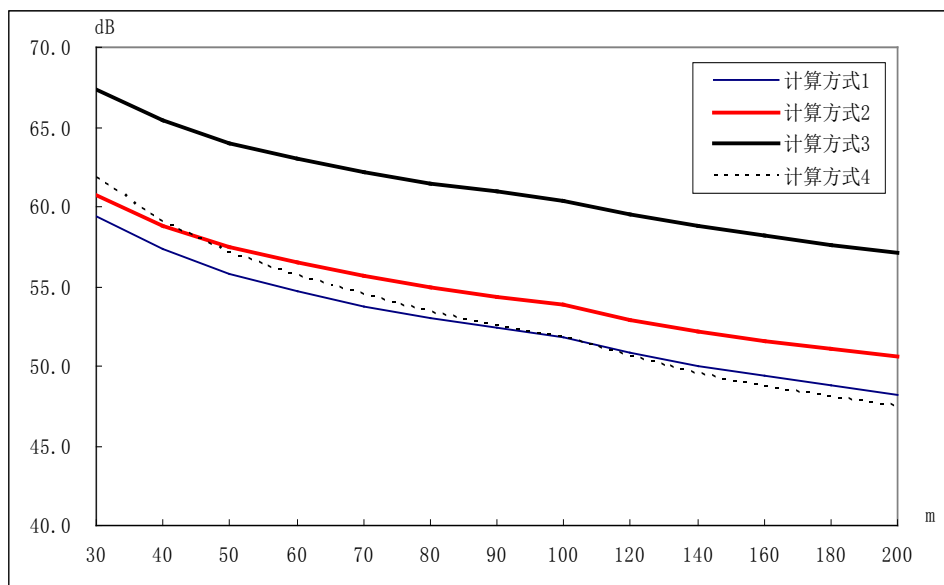
附图 1、交通噪声按不同计算方式昼间结果比较 (2010 年)
