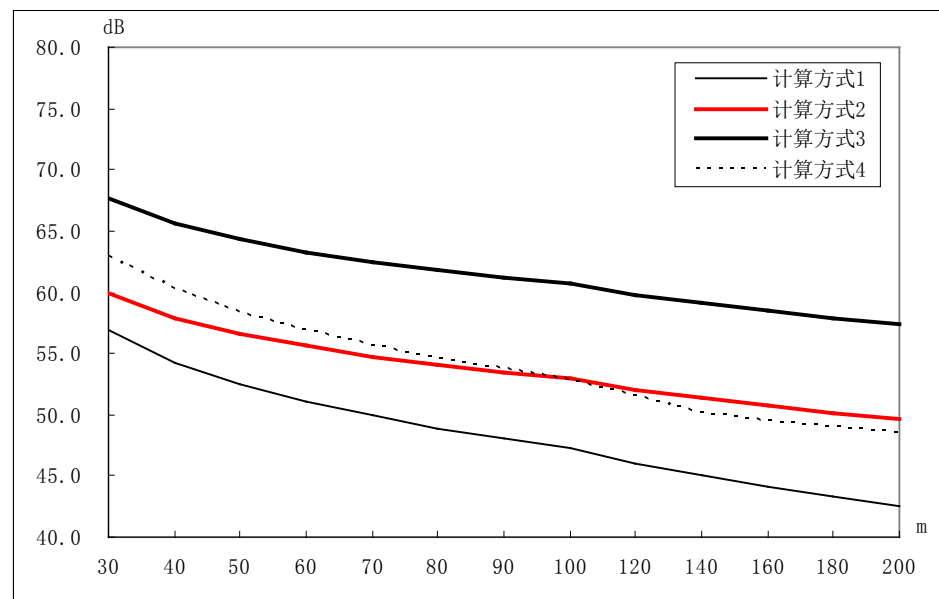
附图 2、交通噪声按不同计算方式夜间结果比较 (2014 年)
