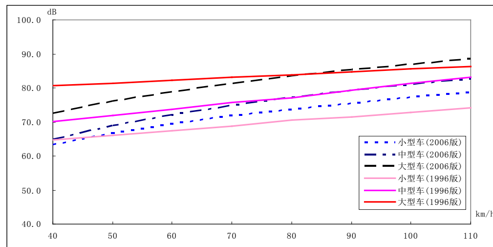
图 2、平均车速与平均辐射声级的关系
