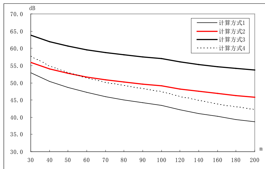
附图 2、交通噪声按不同计算方式夜间结果比较 (2010 年)
