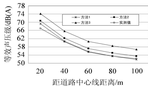
图5 留仙大道噪声预测与实测对比图
