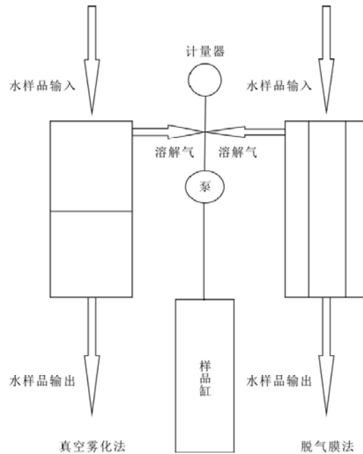
图 B2-1 真空雾化法与脱气膜法原理图
