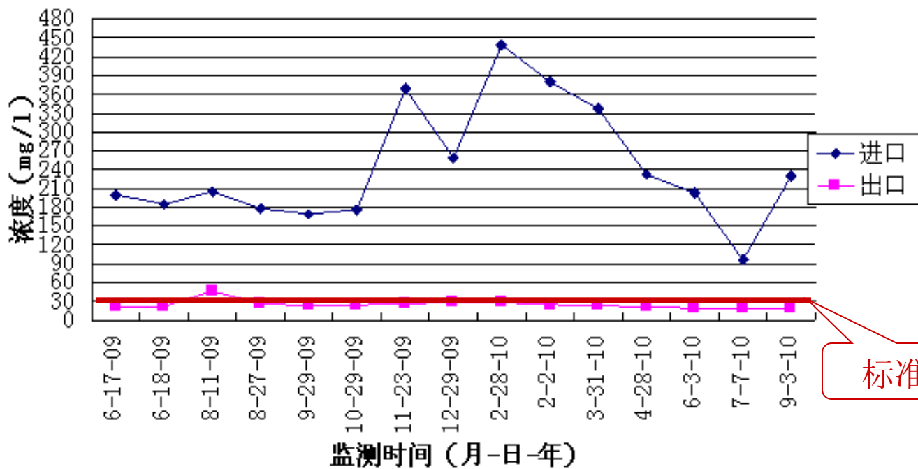
马灌污水处理厂SS监测数据
