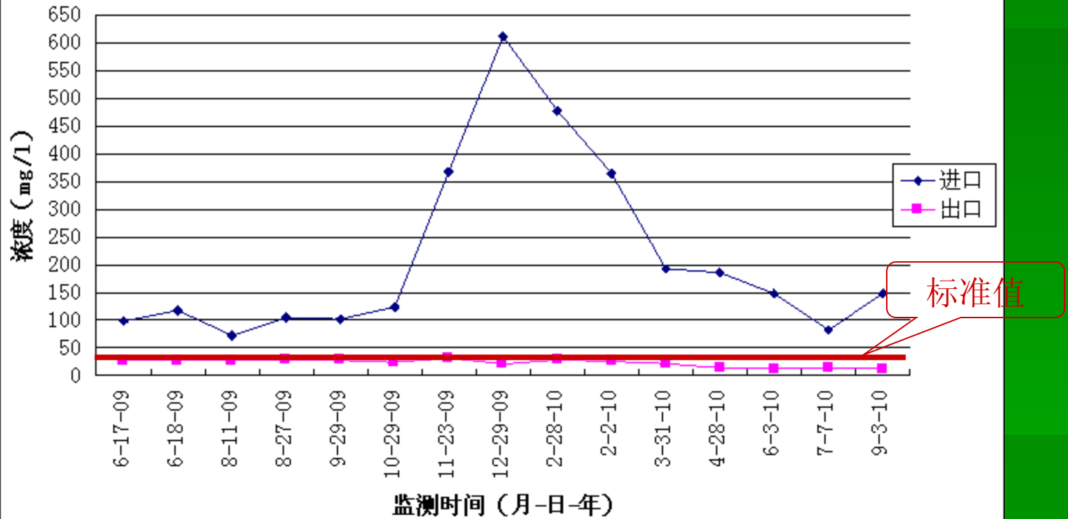
马灌污水处理厂BOD5监测数据
