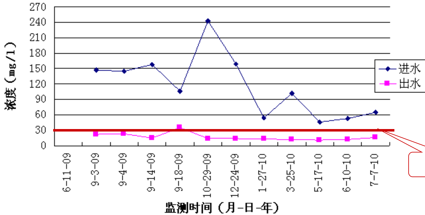
白羊污水处理厂SS监测数据
