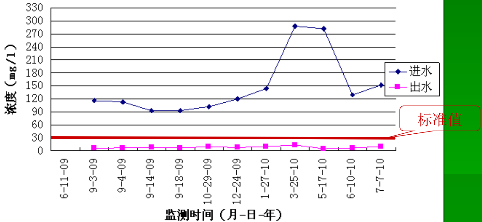
白羊污水处理厂BOD5监测数据
