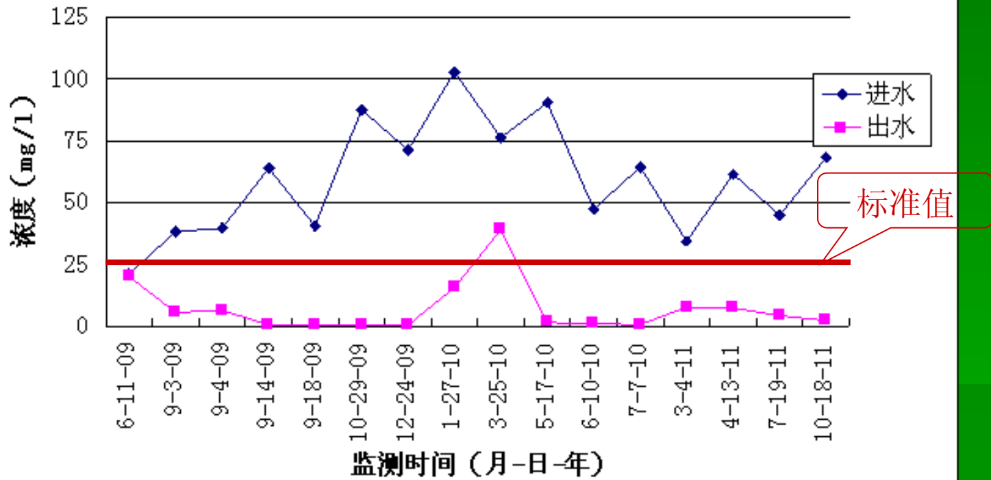
白羊污水处理厂NH 3 -N监测数据
