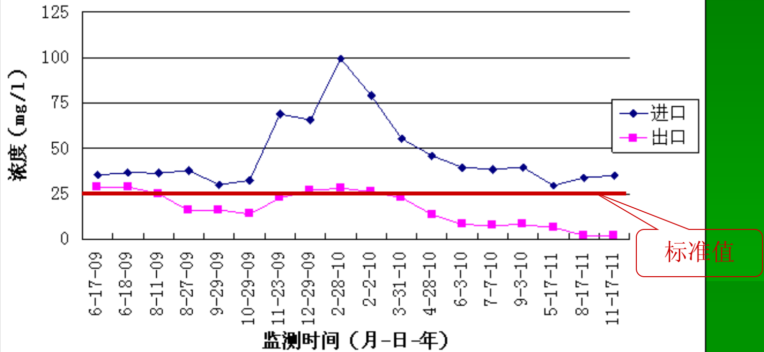
马灌污水处理厂NH 3 -N监测数据
