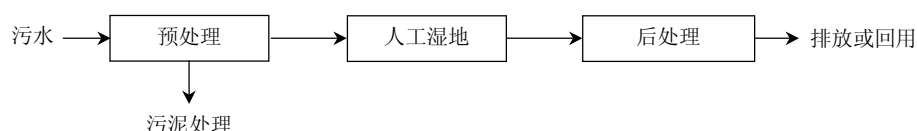
图 1 工程接纳城镇生活污水或与生活污水性质相近的其他污水的工艺流程图
