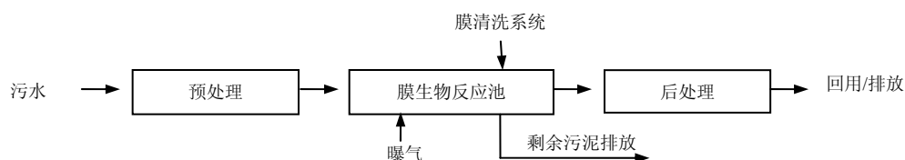
图 1 去除碳源污染物的膜生物法工艺流程图
