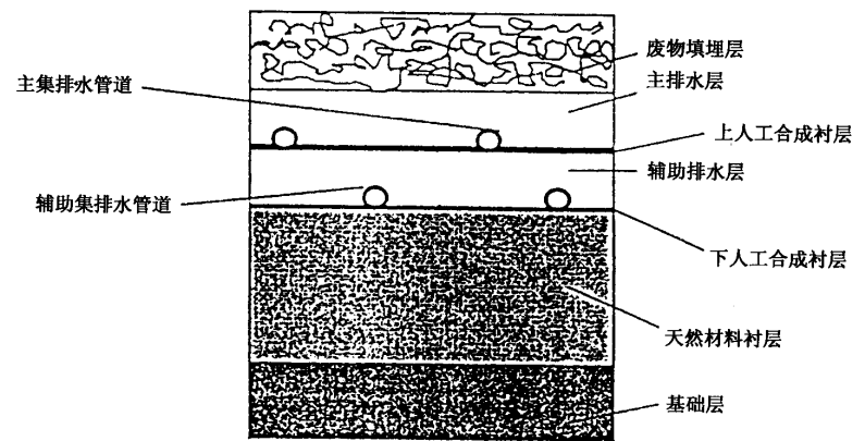
图 1 双层人工衬层示意图
