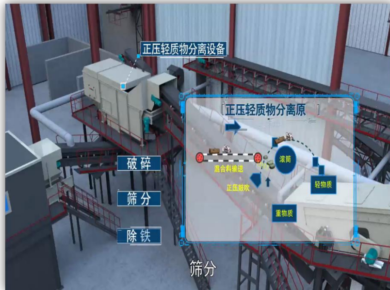
正压鼓吹式除杂
