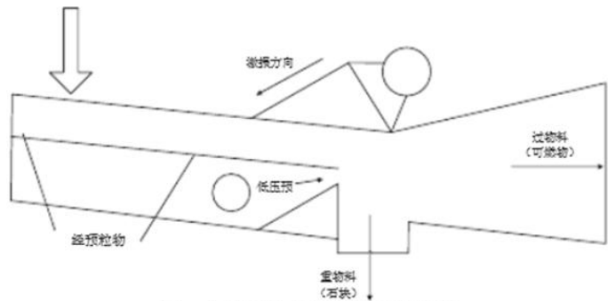
图1 振动风选机工作原理示意图
