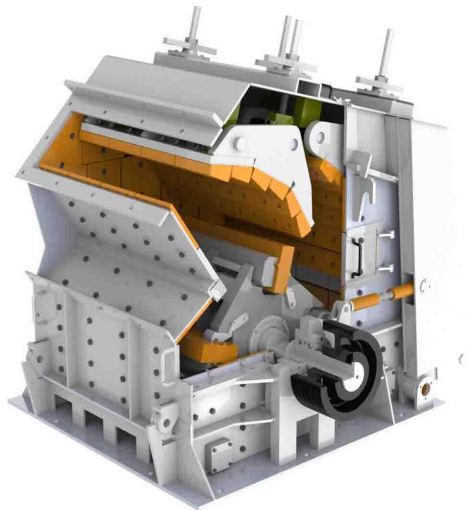
反击式破碎机
