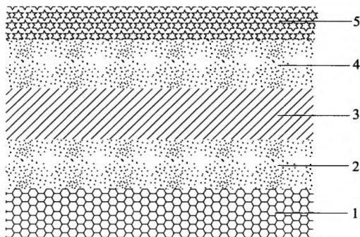
图 13.2.3 黏土覆盖系统示意图
