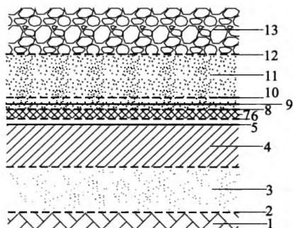
图 8.2.6 库区底部双层衬里结构示意图
