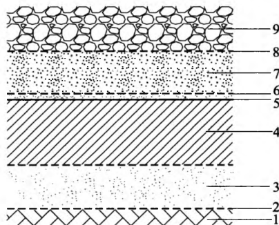
图 8.2.5 库区底部单层衬里结构示意图
