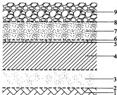
图 8.2.4-1 库区底部复合衬里(HDPE 膜+黏土)结构示意图
