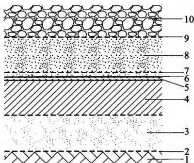
图 8.2.4-2 库区底部复合衬里(HDPE 土工膜+GCL)结构示意图
