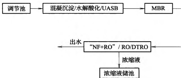
图 2 “预处理+生物处理+深度处理”典型流程
