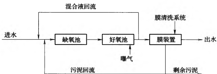
图 1 A/O 工艺流程
