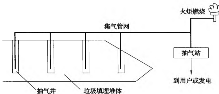
图4 主动导气示意图
