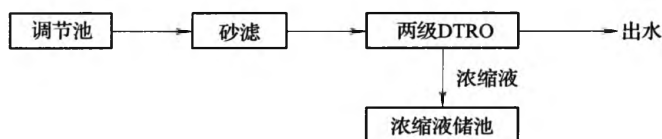
图3 “预处理+深度处理”典型工艺流程
