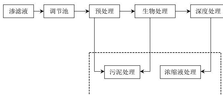
图 1 常规工艺流程图
