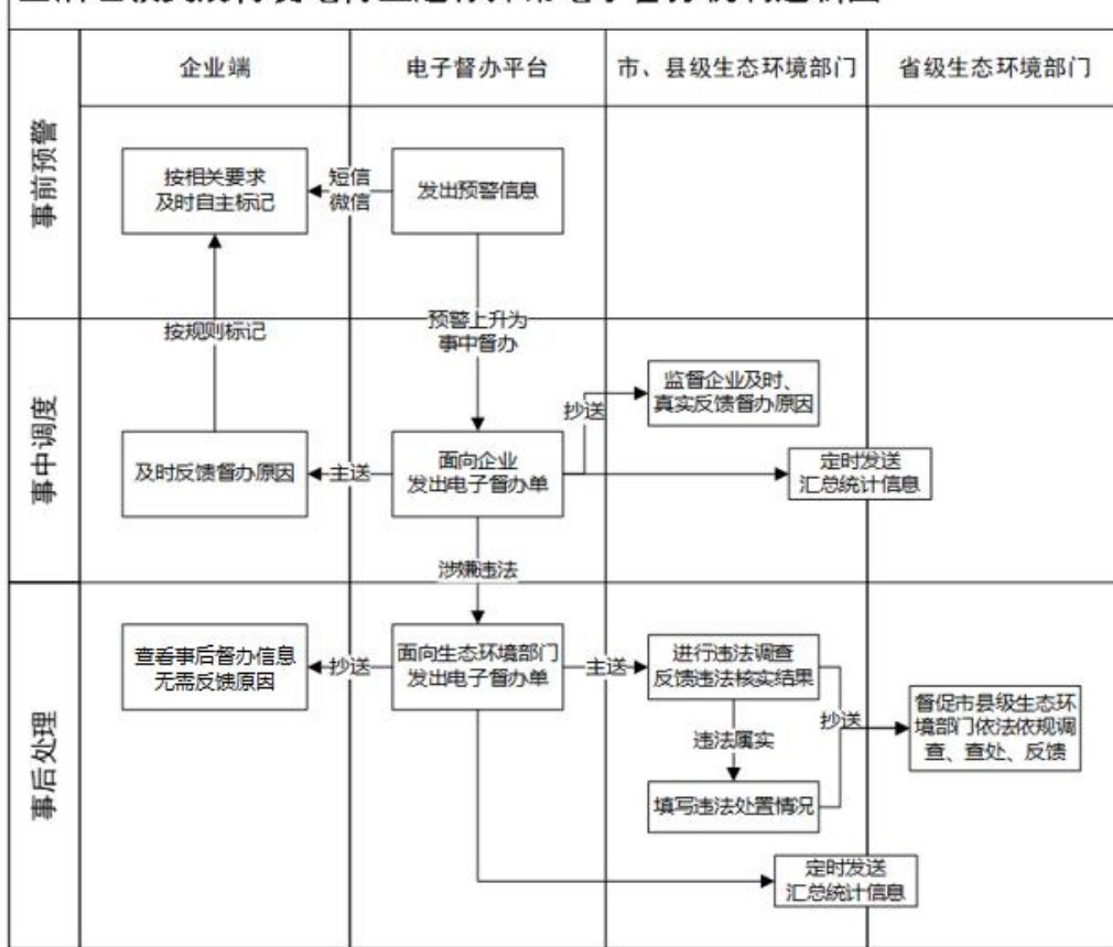
生活垃圾焚烧发电行业超标异常电子督办机制逻辑图
