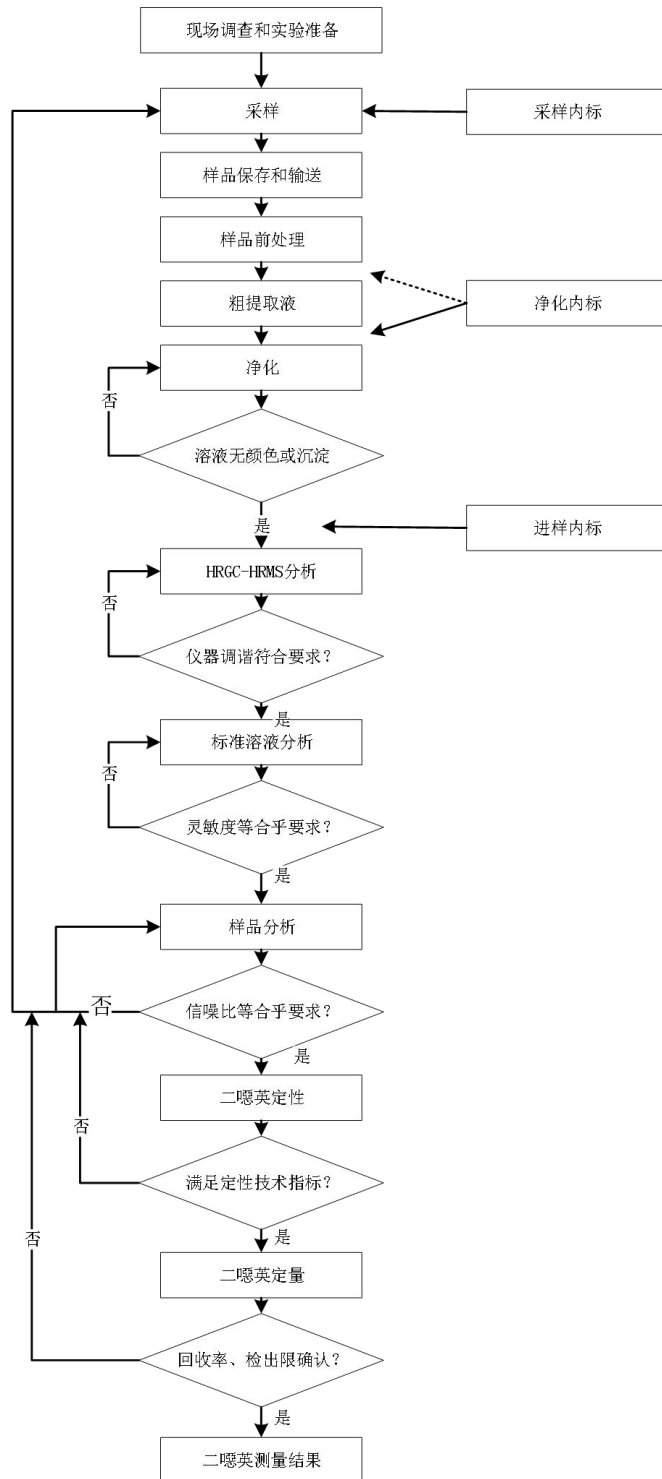
图 C.1 二噁英类监测基本流程图
