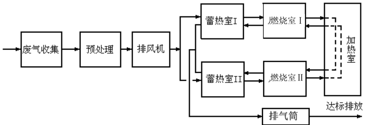
图 2 蓄热催化燃烧工艺流程
