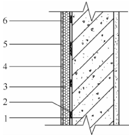
图 5.2.5-1 热桥部位保温处理的基本构造示意
