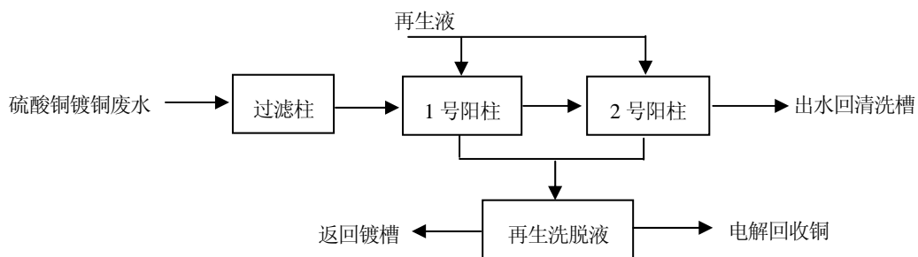
图 15 离子交换处理硫酸铜镀铜废水基本工艺流程
