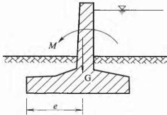
图 5.4.3 防火堤抗倾覆验算简图
