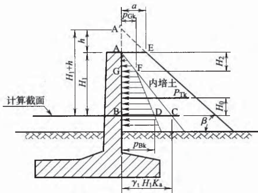
图 5.2.3 内培土压力计算示意图
