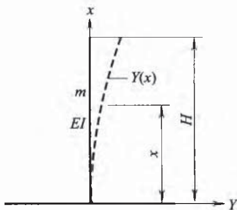
图2 振型函数曲线
