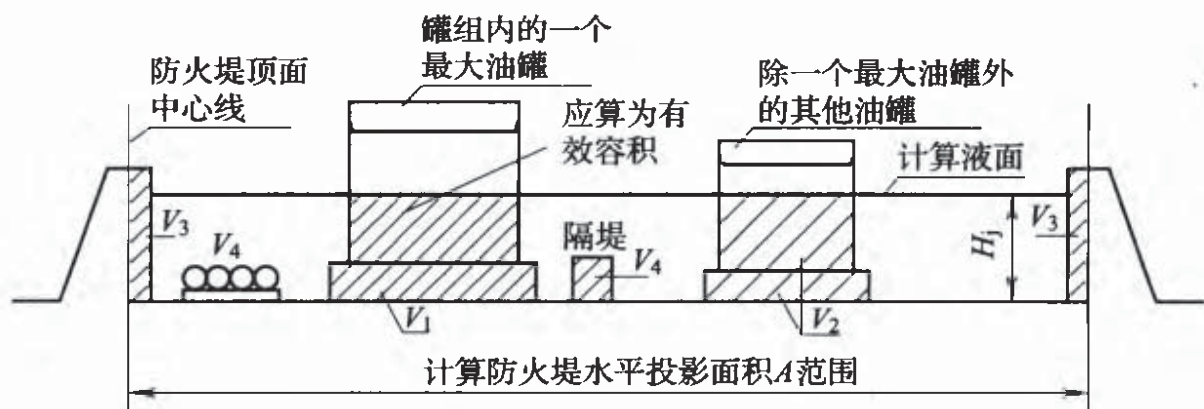
图 1 防火堤有效容积计算示意
