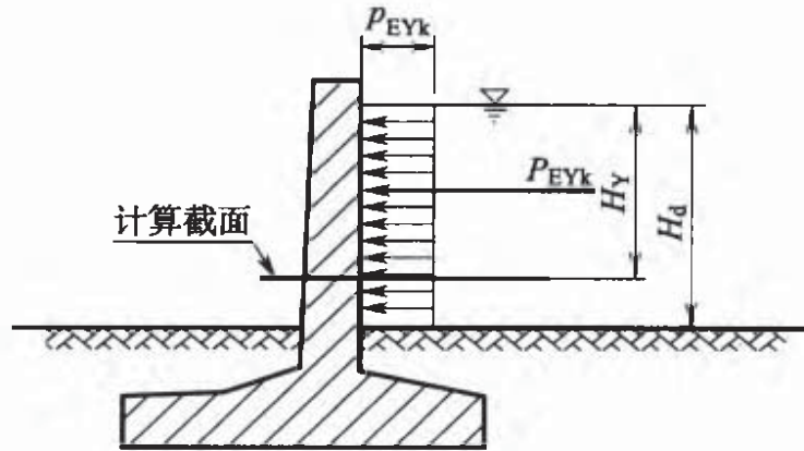
图 5.2.5 水平动液压力计算示意图
