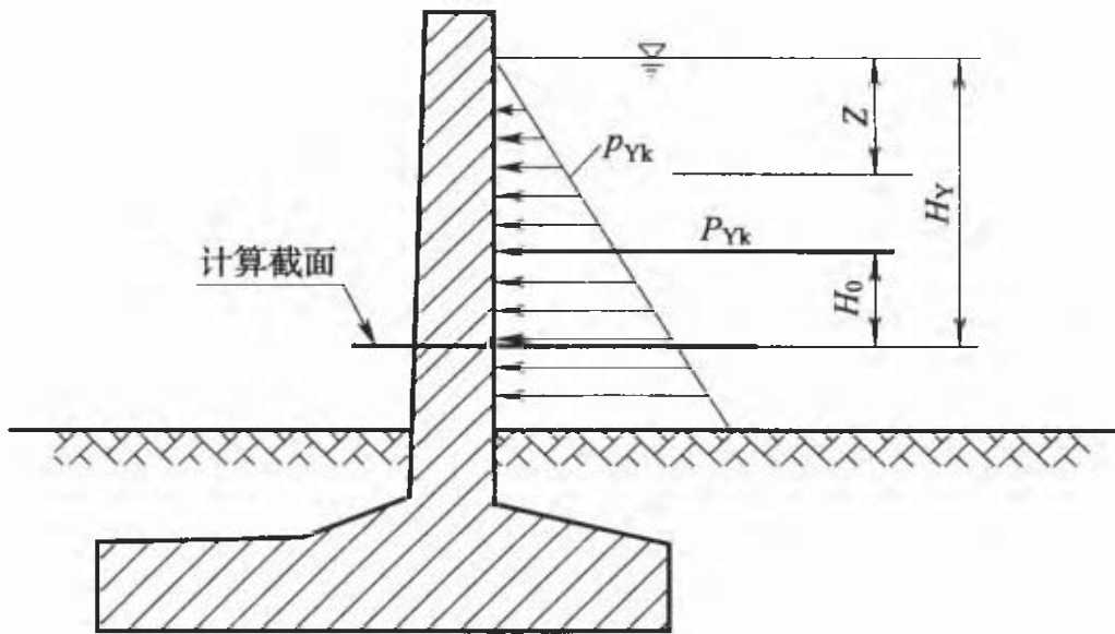
图 5.2.2 静液压力计算示意图
