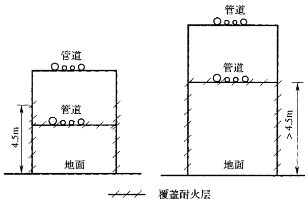
图 6 钢管架 I
