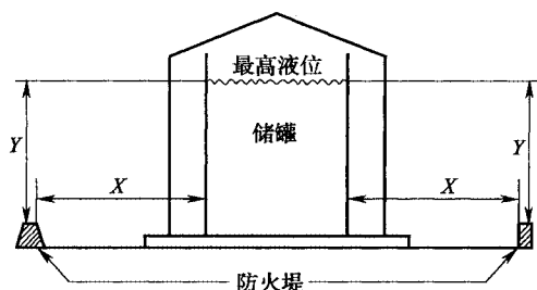
图 6.3.6 单防罐至防火堤内顶角线的距离
