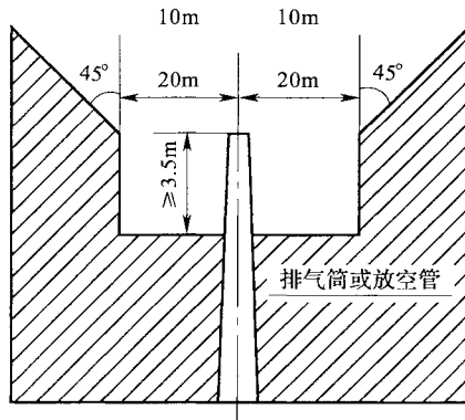
图 5.5.11 可燃气体排气筒、放空管高度示意图
