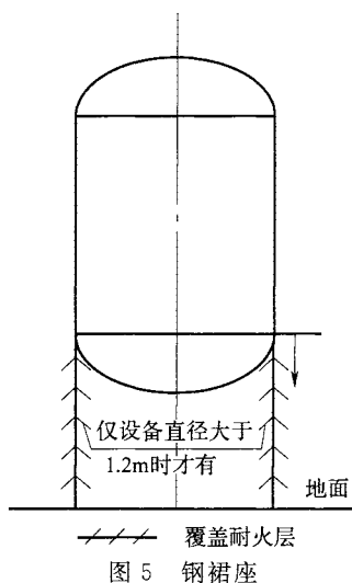
图 5 钢裙座
