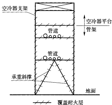
图 7 钢管架 II
