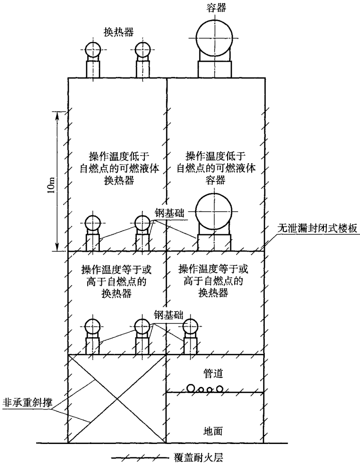
图 3B 操作温度等于或高于自燃点的可燃液体设备上方,布置操作温度低于自燃点的甲、乙、丙类可燃液体设备的构架
