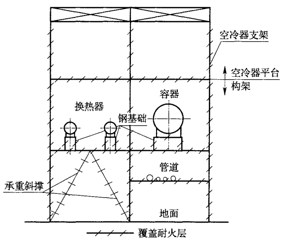
图 3A 上部设有空气冷却器的构架
