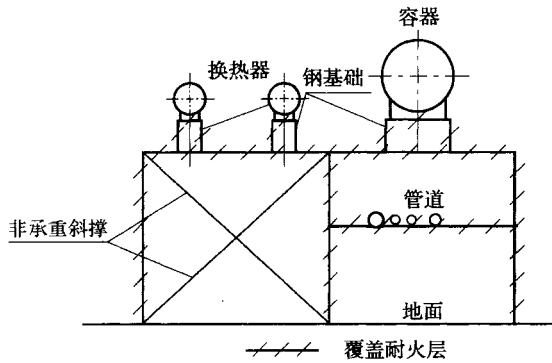
图 1 单层构架
