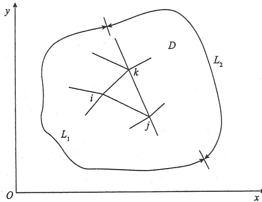
图 F. 1 三角形单元示意图
