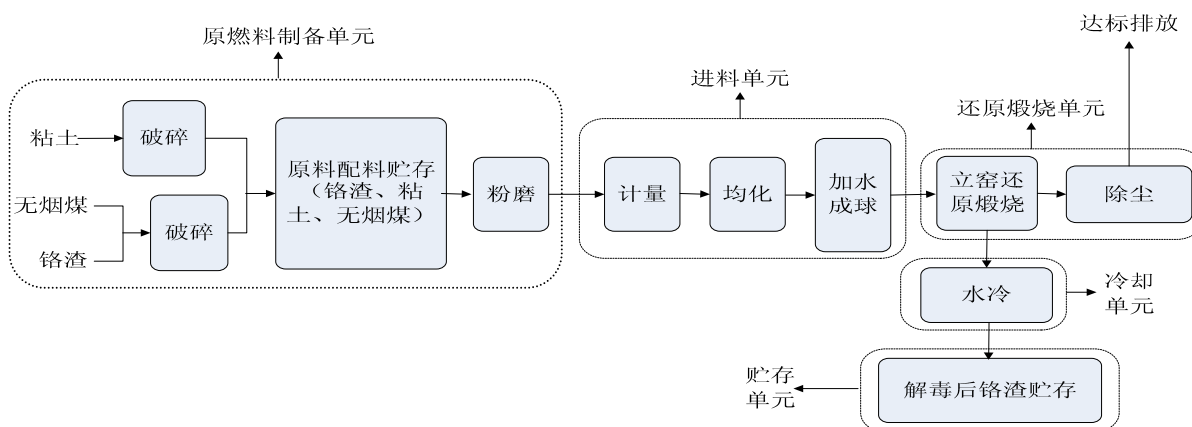
图 2 立窑干法解毒工艺流程图
