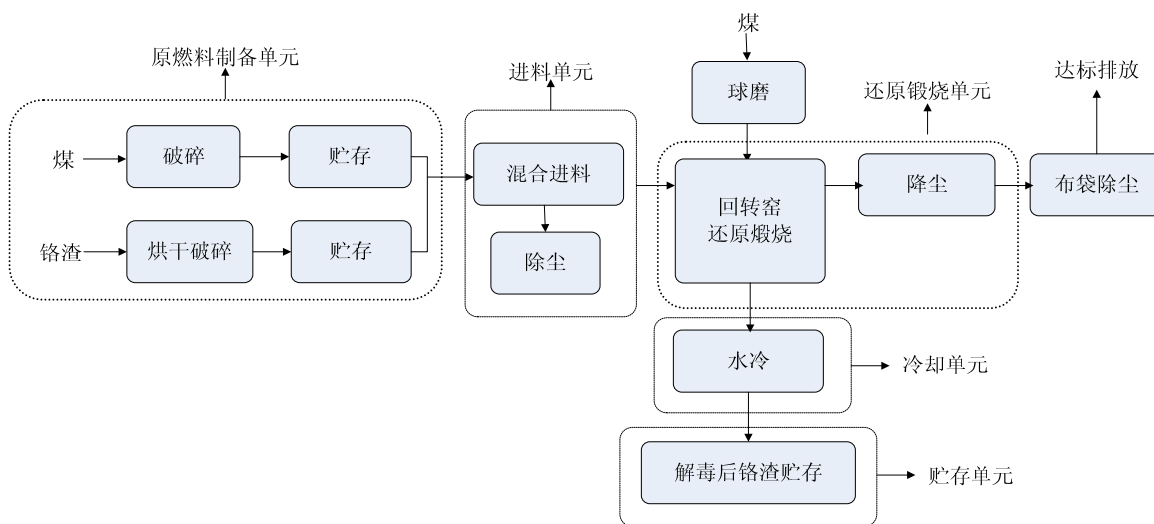
图 1 回转窑干法解毒工艺流程图
