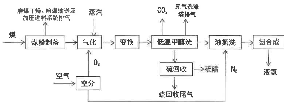
图 25-2 干煤粉气流床气化工工艺合成氨生产工艺流程图
