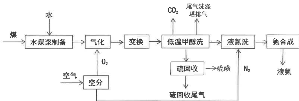
图 25-1 水煤浆气流床气化工工艺合成氨生产工艺流程图
