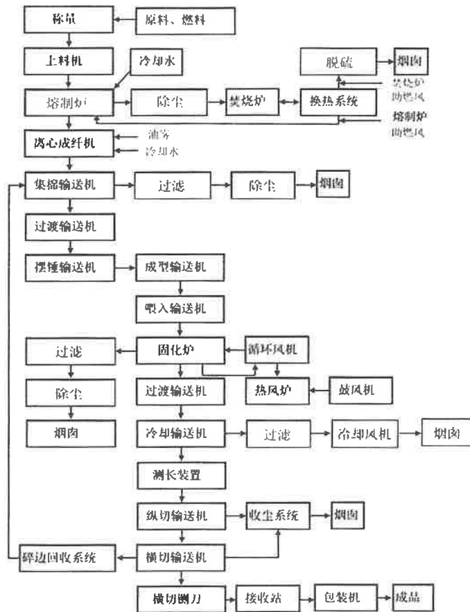
图 20-1 岩棉生产典型工艺流程图
