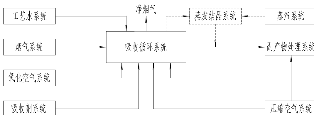
图 1 氨法烟气脱硫工艺流程示意图
