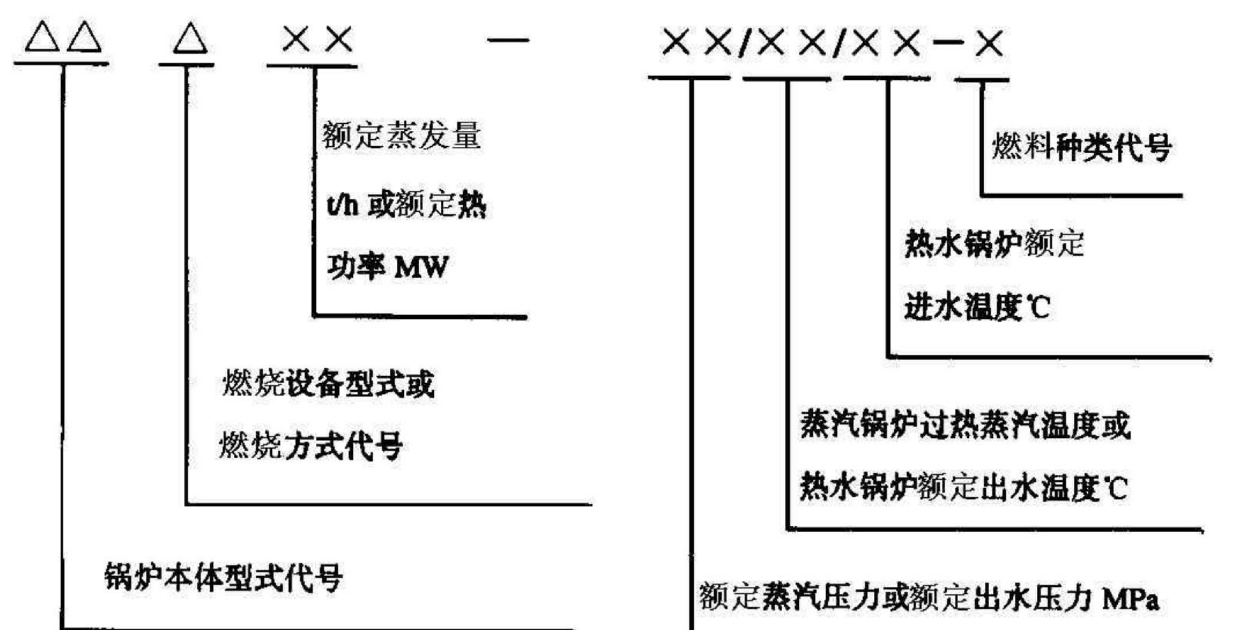
图1 工业锅炉产品型号组成示意图
