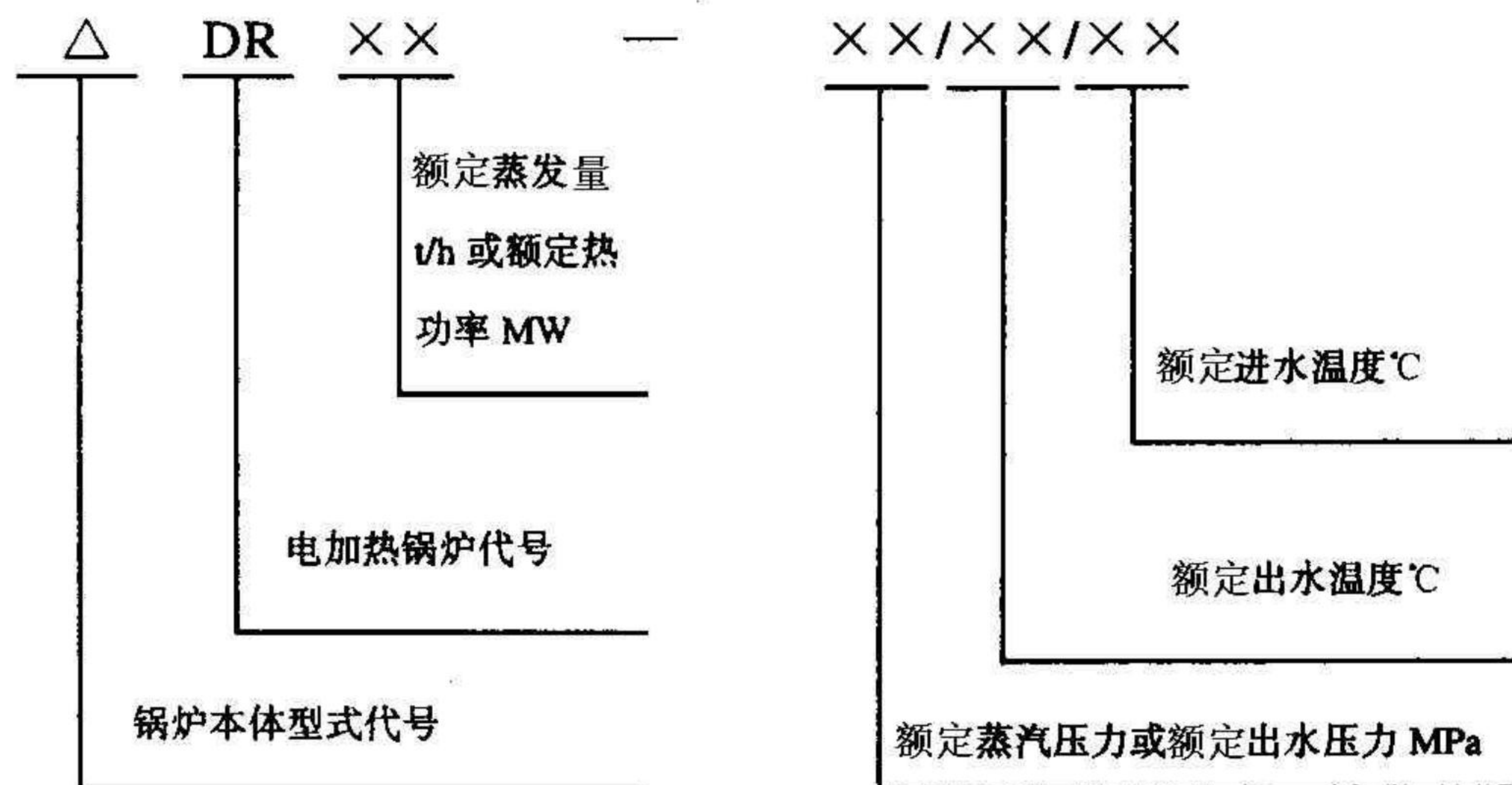
图2 电加热锅炉产品型号组成示意图
