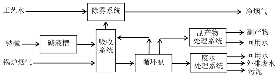
图 6 钠碱法烟气脱硫典型工艺流程
