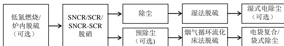
图 1 煤粉锅炉及循环流化床锅炉烟气治理工艺流程
