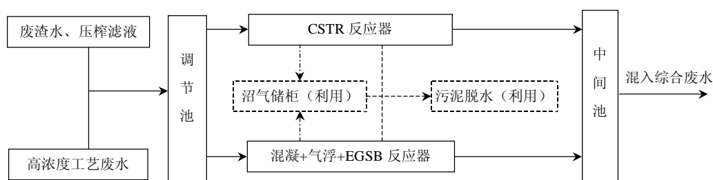
图 4 高浓度工艺废水一级厌氧发酵处理工艺流程图
