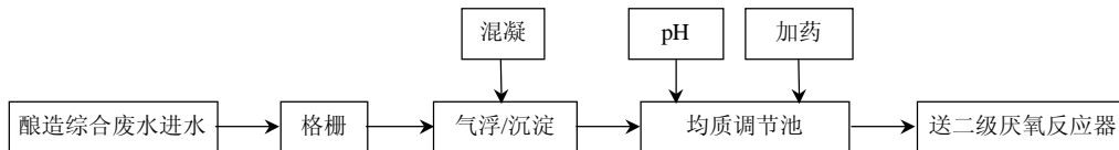
图 5 综合废水前处理系统工艺流程图
