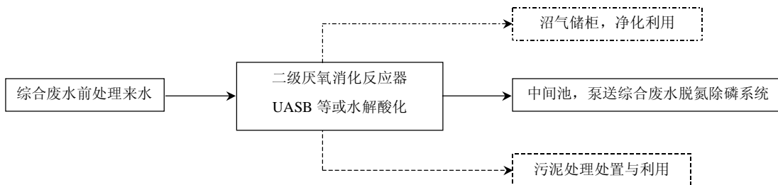
图 6 二级厌氧消化处理系统工艺流程图
