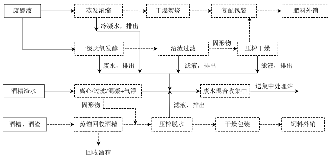
图2 固形物回收处理工艺流程图
