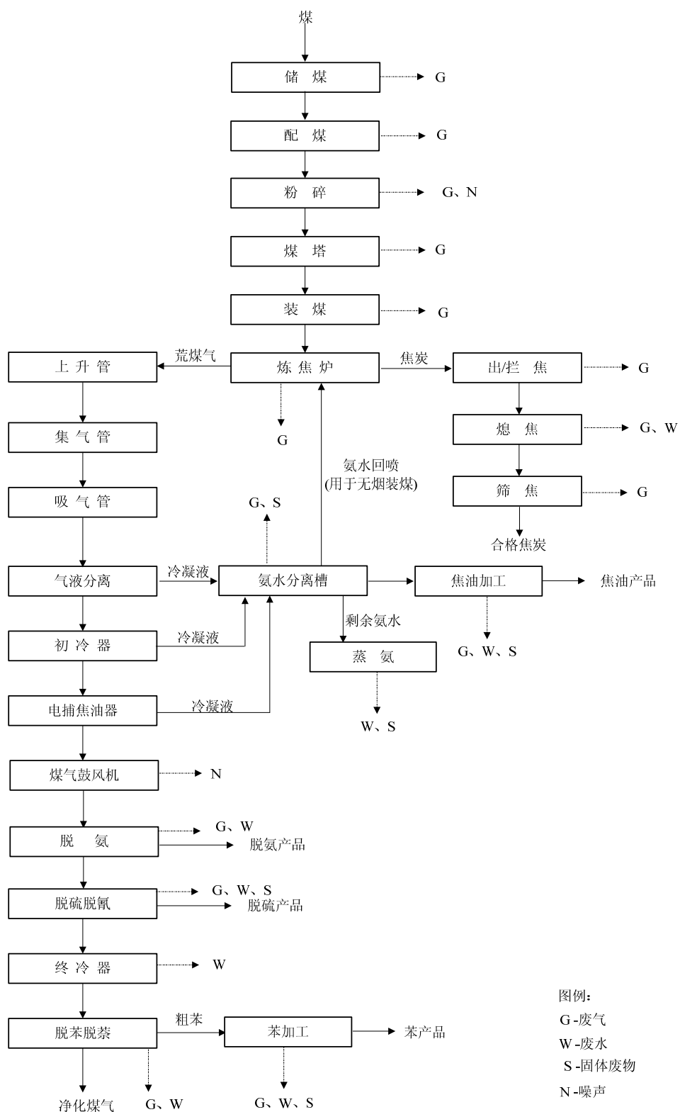
图 1 焦化工序流程及产污环节
