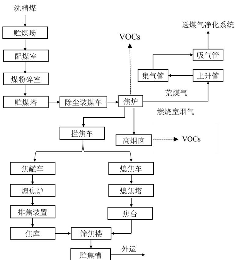
图 1-1 炼焦生产工艺流程与 VOCs 排放环节图
