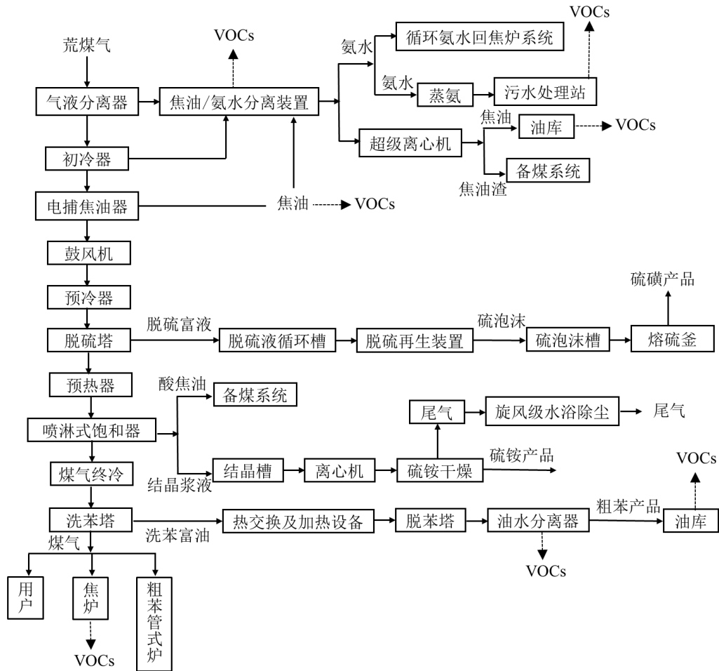
图 1-2 焦炉煤气净化典型工艺与 VOCs 排放环节图
