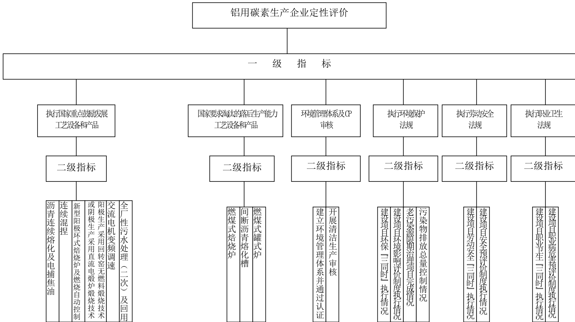
图 11 铝用碳素生产企业定性评价指标体系框架
