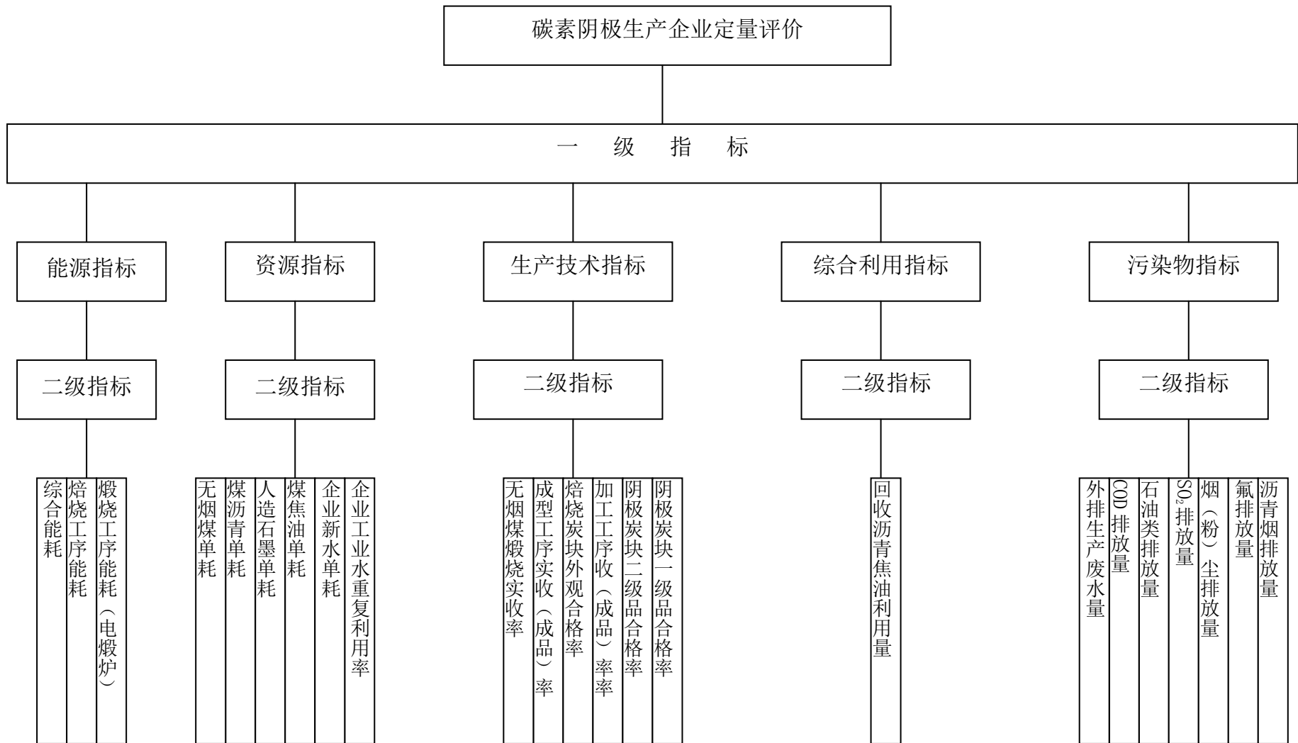
图 10 碳素阴极生产企业定量评价指标体系框架
