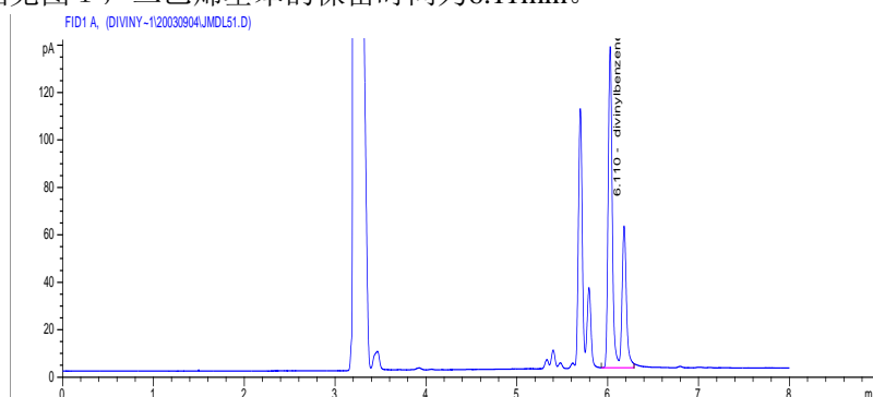
图 1 色谱分离图
