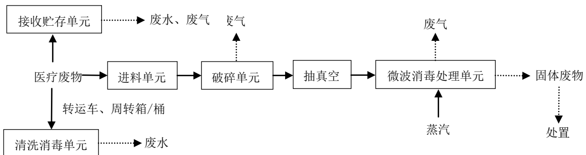
图 2 微波与高温蒸汽组合消毒处理工艺流程
