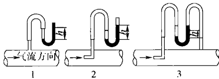
图 19 用 U 形管压力计测定风压
