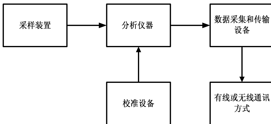
图 1 点式连续监测系统组成示意图
