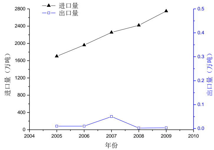
图 8: 2005-2009 年全国废纸进出口量
