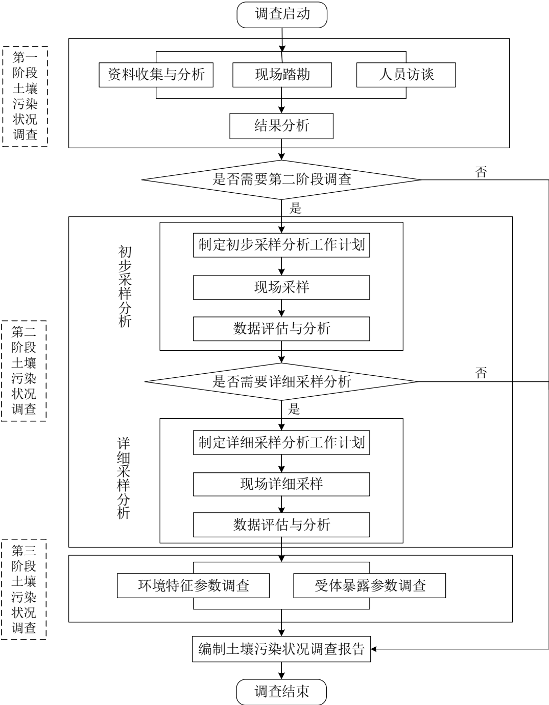
图1 建设用地土壤污染状况调查工作程序
