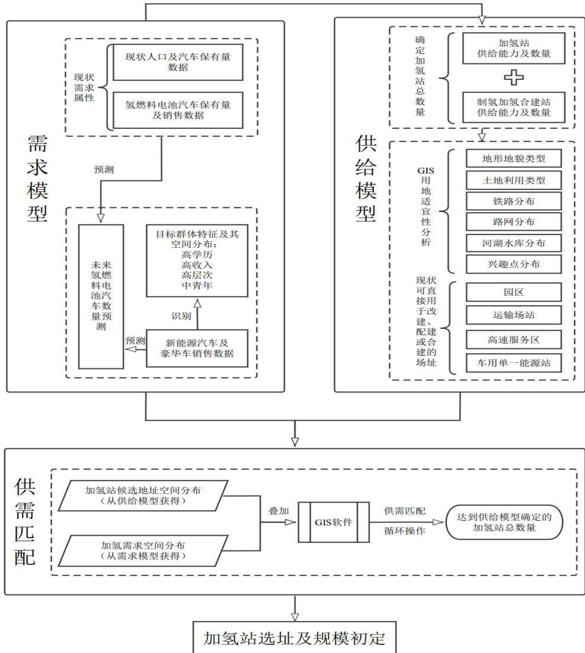
图2 需求与供给技术流程简图
