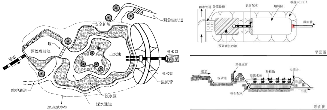
图 2-12 表面流雨水湿地和小型潜流雨水湿地构造示意图
