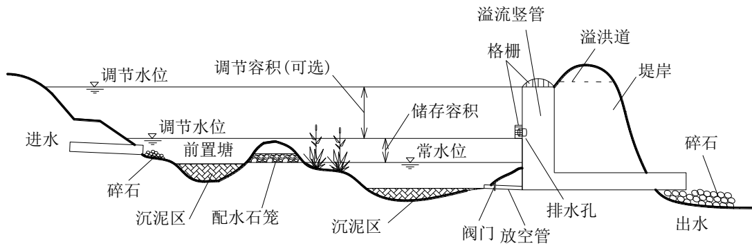
图 2-10 湿塘典型构造示意图
