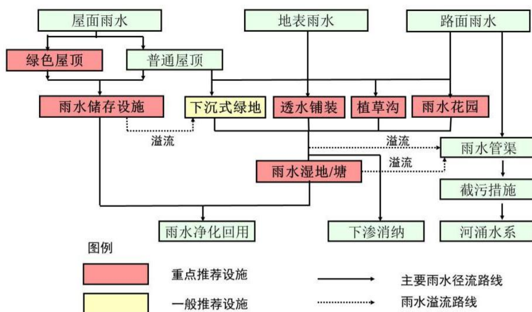
图 6-2 建筑与小区低影响开发雨水系统典型流程（推荐）
