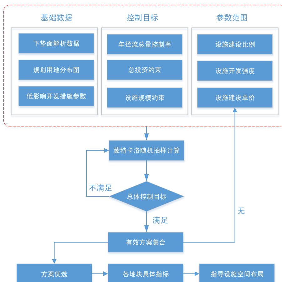
图 3-1 控制指标的模拟分解与优化流程图
