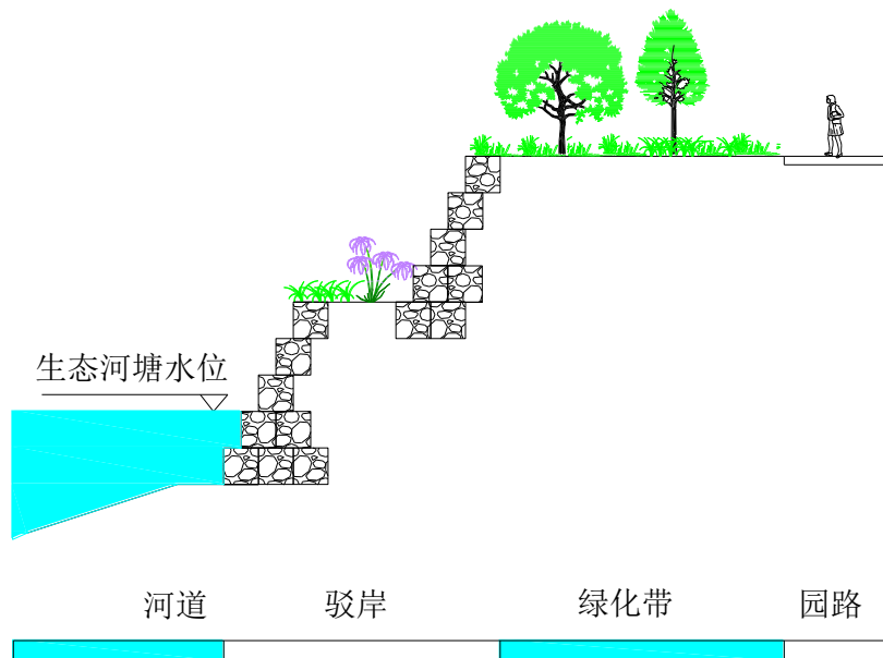
图 2-21 生态型台阶种植驳岸 2
