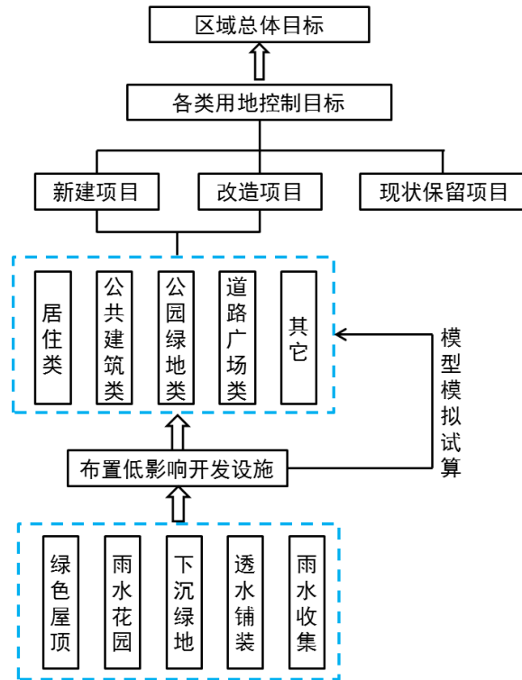
图 3-4 年径流总量控制率目标分解流程
