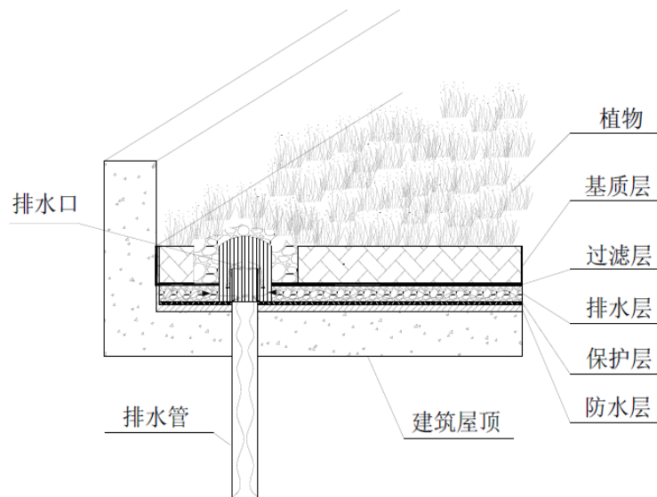
图 2-15 绿色屋顶构造图
