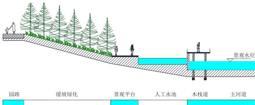
图 2-23 生态型亲水驳岸 1
