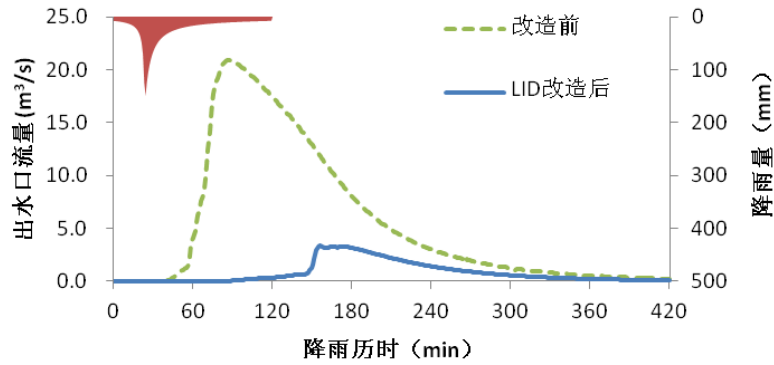
图 3-11 LID 方案实施前后出水口流量过程线图
