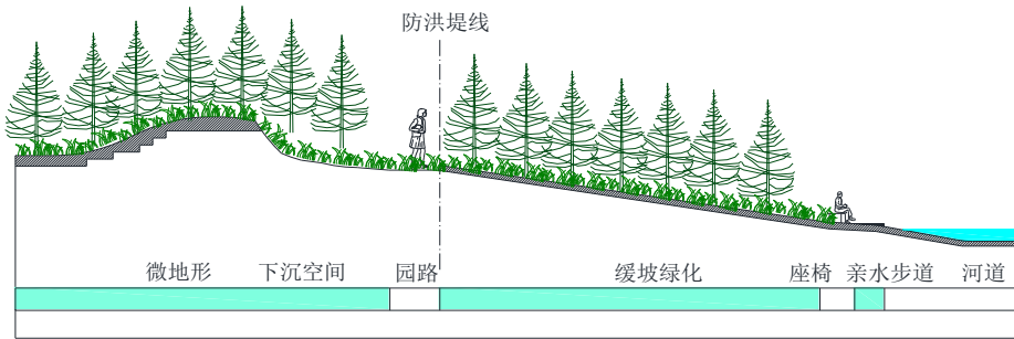
图 2-22 生态型人工草坡驳岸
