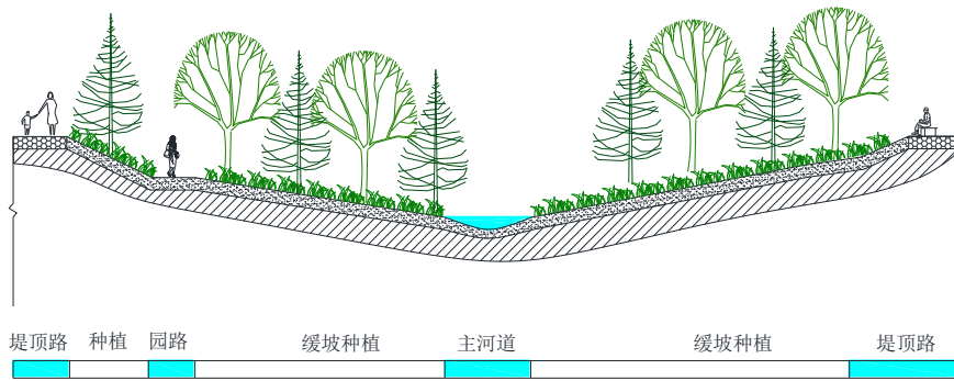
图 2-25 生态型自然林地驳岸
