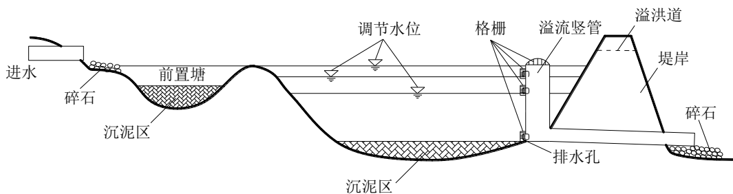
图 2-14 调节塘典型构造示意图
