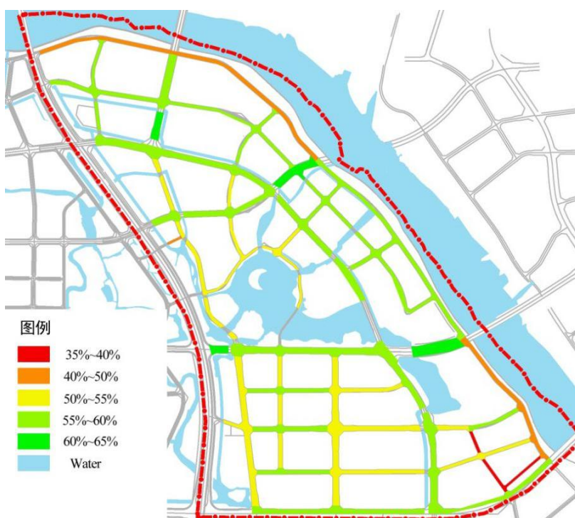
图 3-7 市政道路年径流总量控制率控制指标分布图
