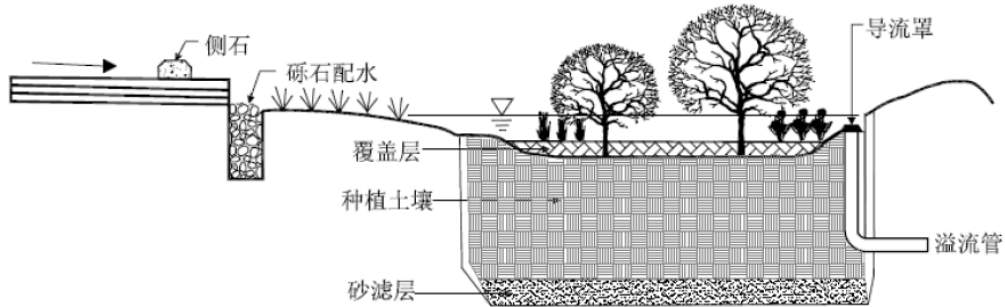
简易型雨水花园结构图
