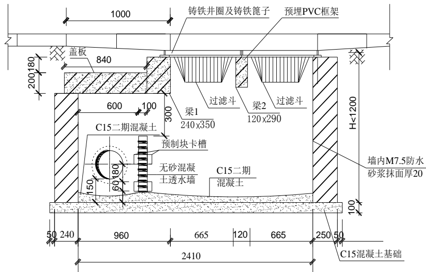
图 2-16 典型环保型雨水口构造图
