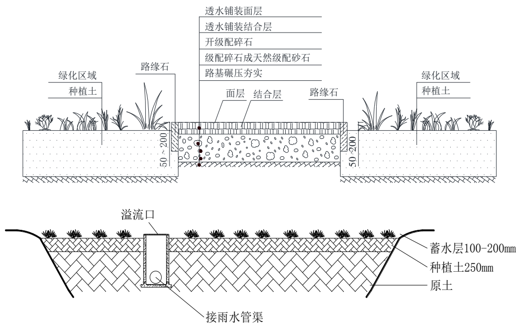
图 2-6 狭义的下沉式绿地典型构造示意图
