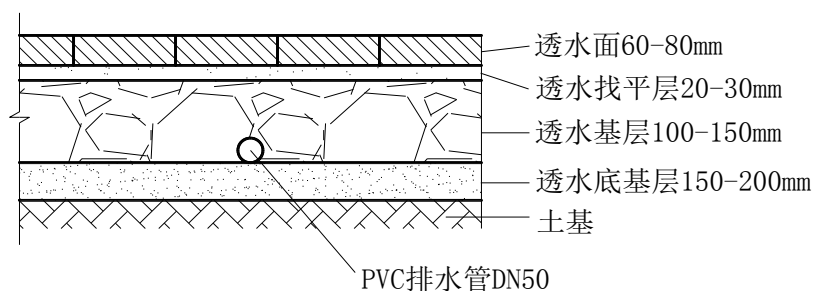
图 2-1 透水砖铺装典型结构示意图
