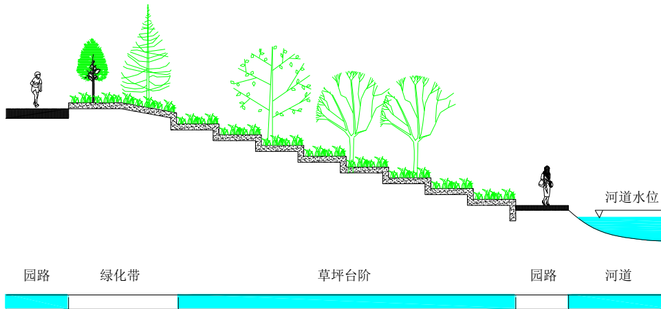
图 2-20 生态型台阶种植驳岸 1
