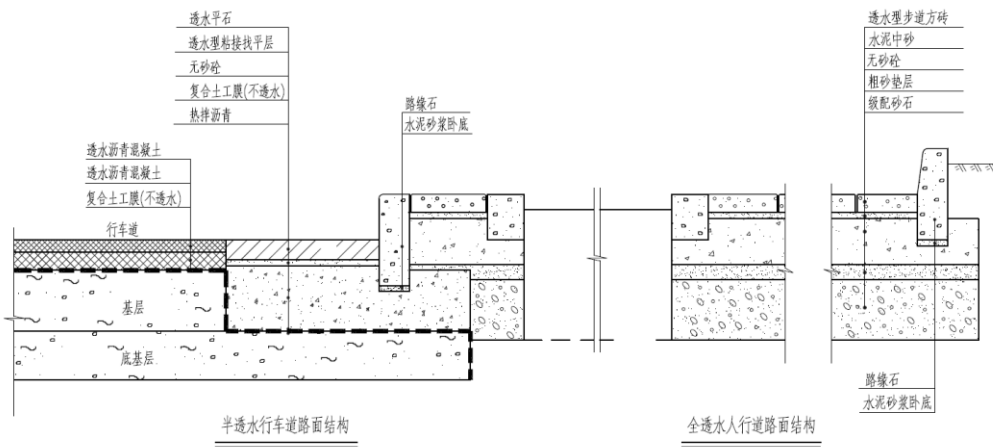
图 2-3 透水铺装路面（二）
