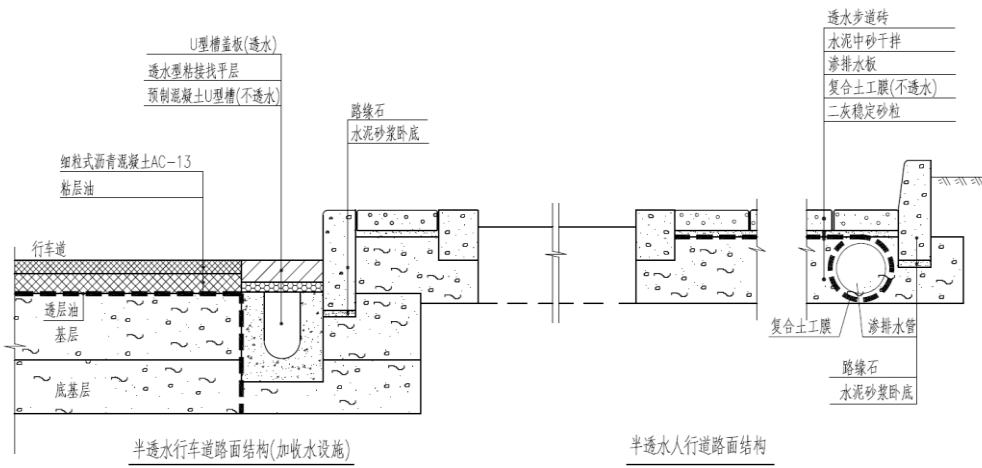
图 2-4 透水铺装路面（三）
