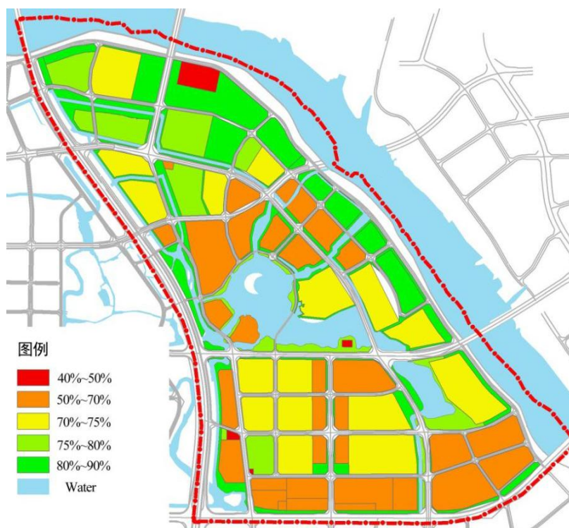
图 3-6 地块年径流总量控制率控制指标分布图
