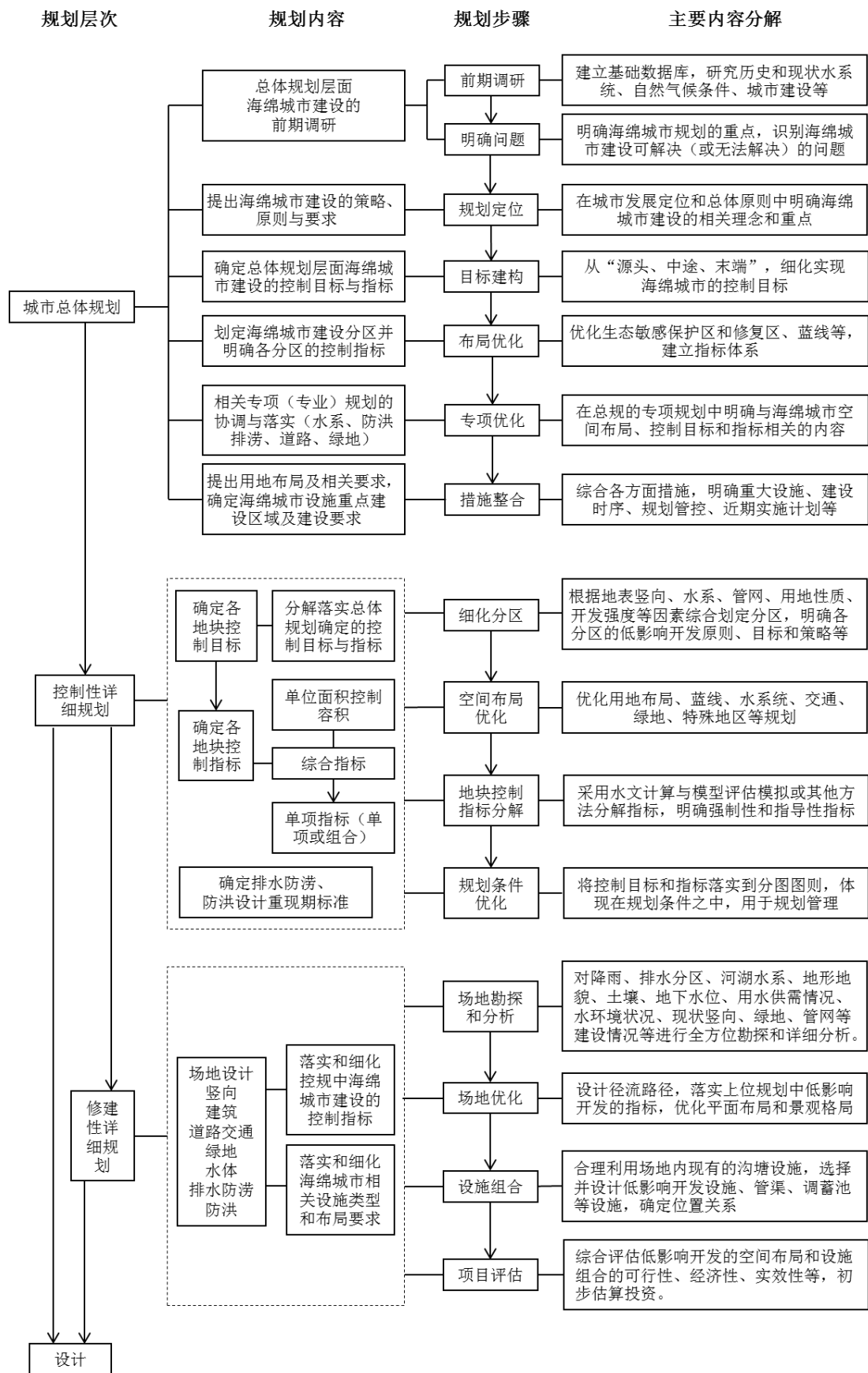
图 5-1 海绵城市专项规划（总规、控规、修规各层面）技术路线图
