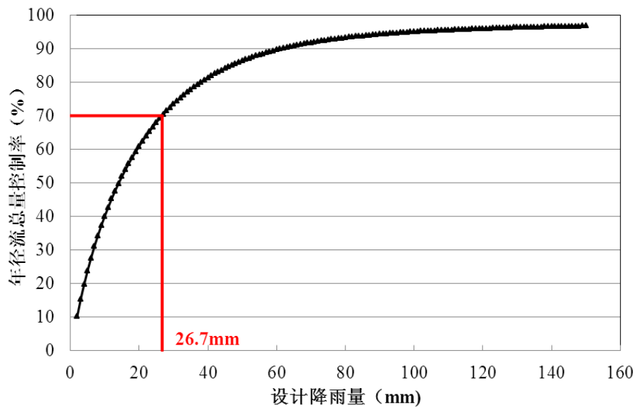
图 4-1 佛山市不同年径流总量控制率对应的设计降雨量
