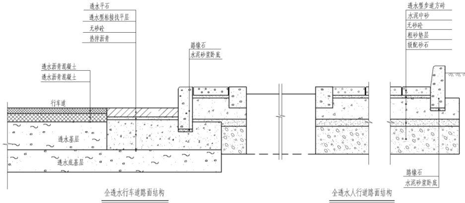
图 2-2 透水铺装路面（一）
