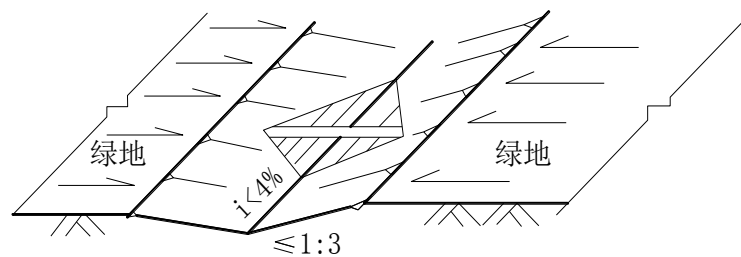
图 2-27 转输型植草沟典型构造图
