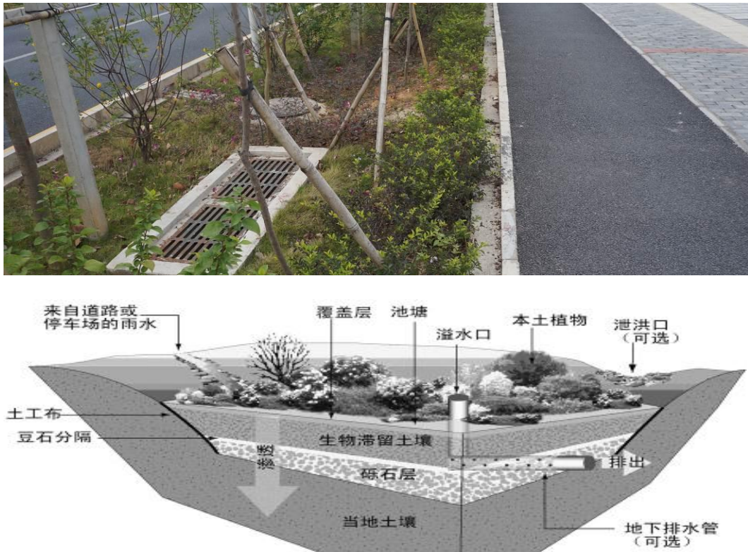
图 2-8 生物滞留设施实景图 and 构造图
