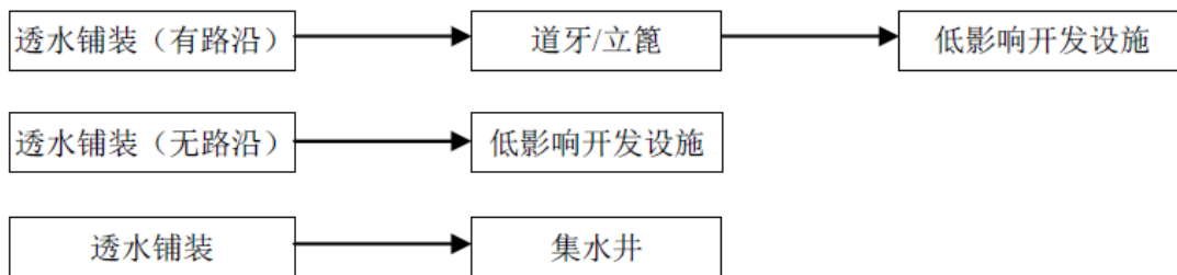
图 2-5 透水铺装溢流设施
