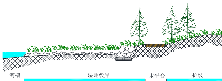
图 2-26 生态型自然湿地驳岸
