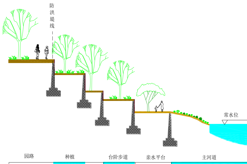
图 2-18 生态型台阶步道驳岸 1
