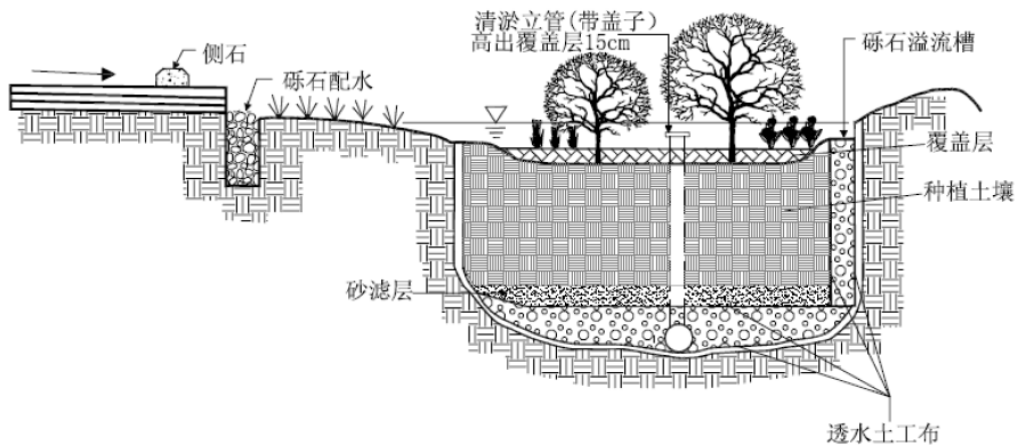
增强型雨水花园结构图
