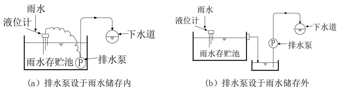
图 2-13 溢流排水方式示意
