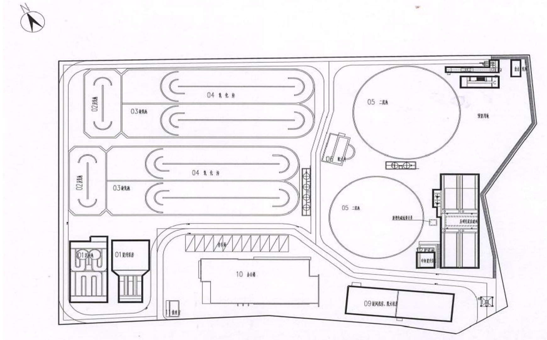
附件 8 项目总平面布置图
