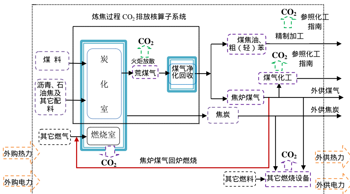
图 1 独立焦化企业温室气体排放核算边界示意图（以常规机焦炉为例）
