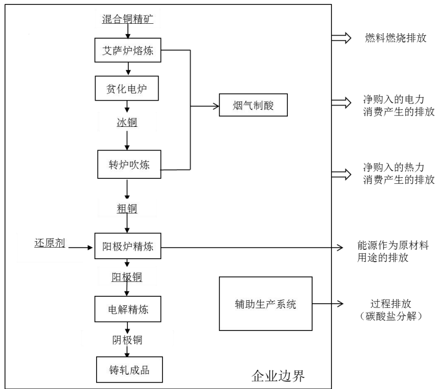
图 1 其他有色金属冶炼和压延加工业企业温室气体核算边界示意图 (以铜冶炼为例)
