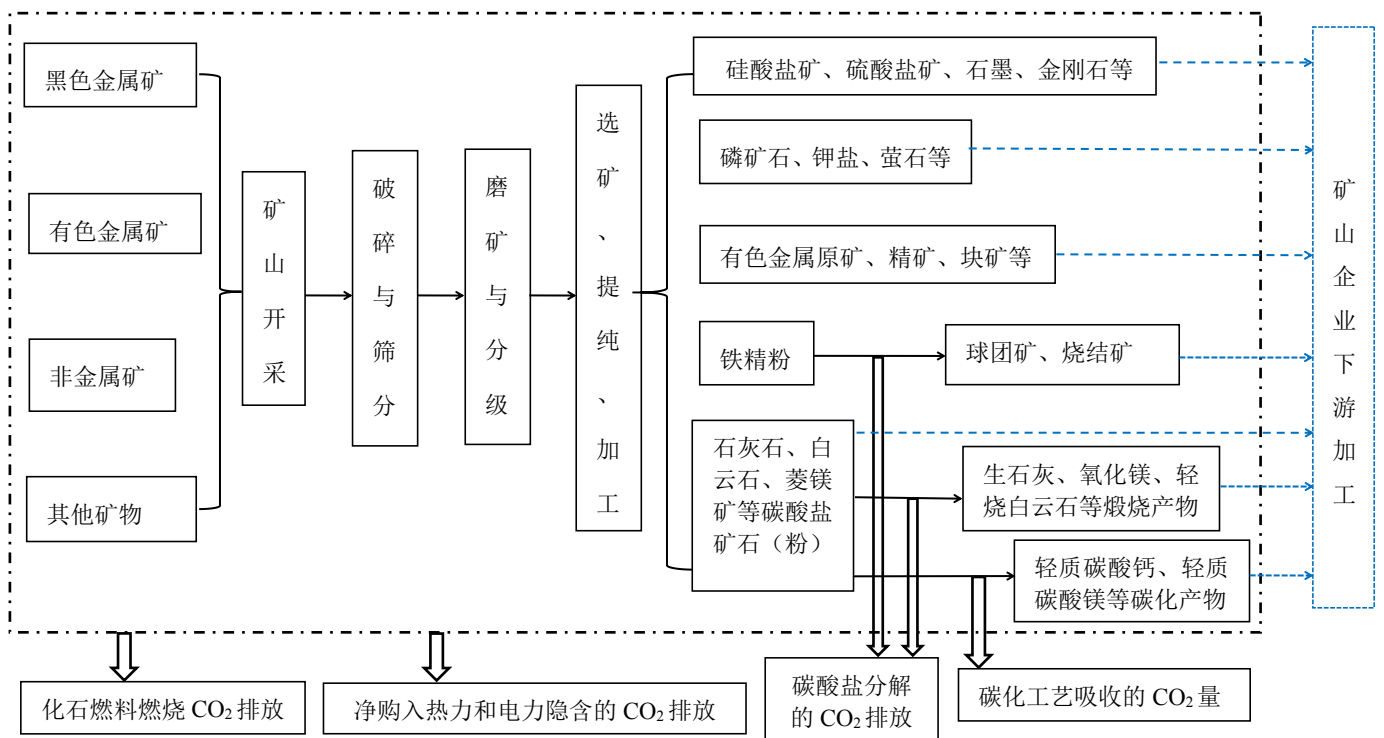
图 1 矿山企业生产工艺流程和温室气体排放源示意图
