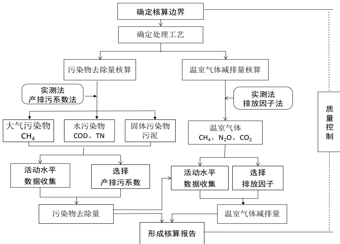
图 1 工作流程
