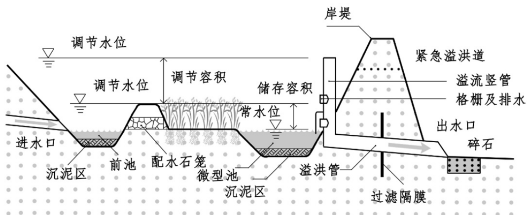
图 5.2.17 湿塘的典型构造示意图
