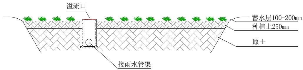
图 5.2.14 下凹式绿地典型构造示意图
