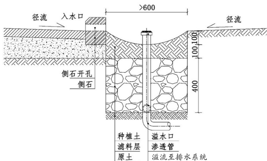
图 5.2.16 植草沟典型构造示意图
