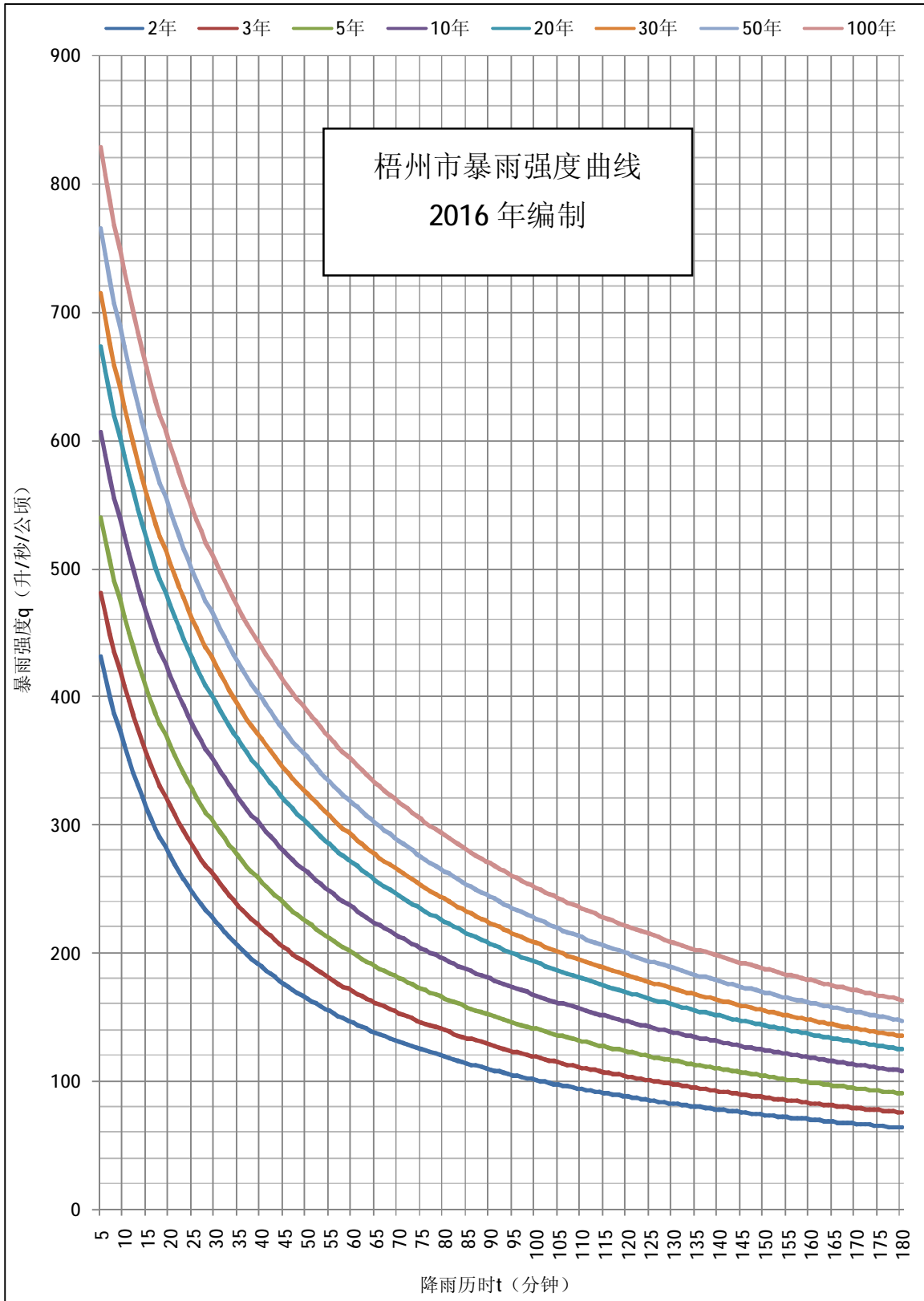
图 1 不同重现期下暴雨强度随历时变化曲线图
