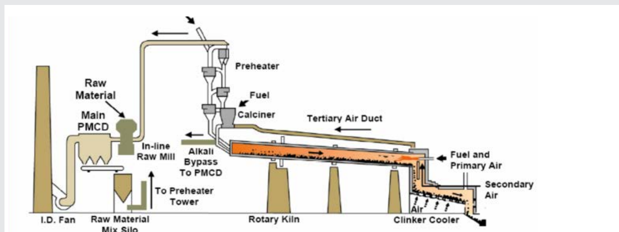
图表 9.4-3 预分解窑系统
