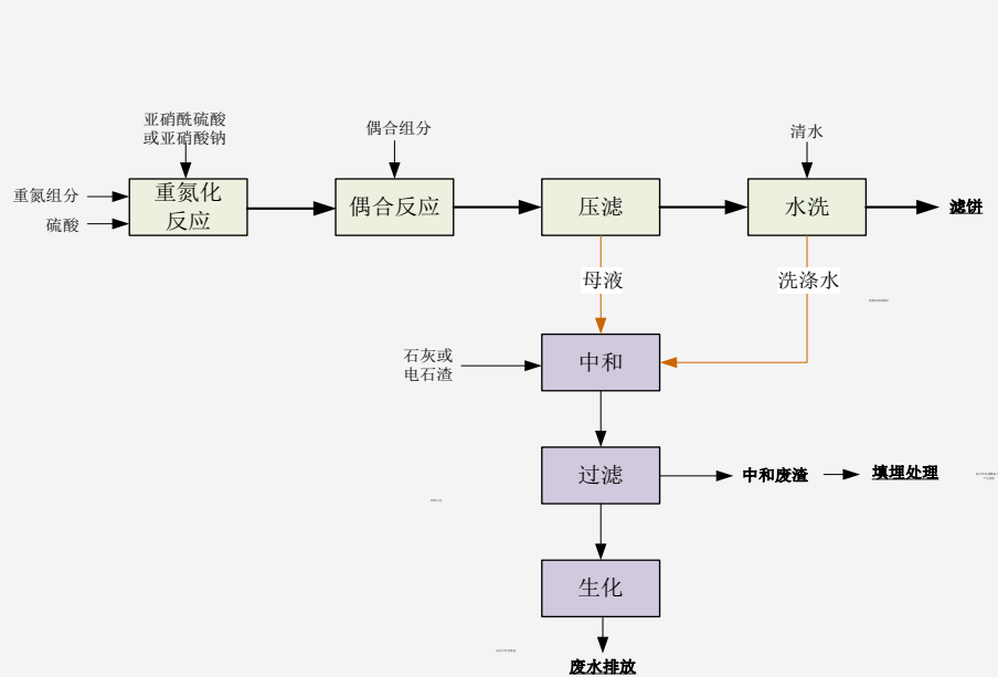
传统分散染料生产及废水处理流程图
