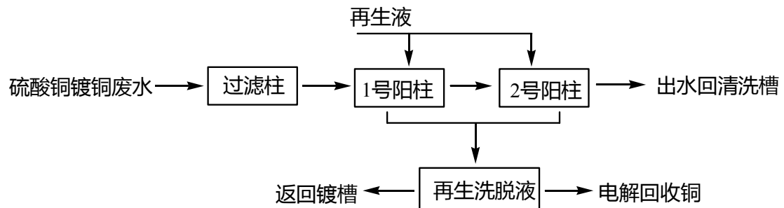
图 4.1-10 离子交换处理硫酸铜镀铜废水基本工艺流程
