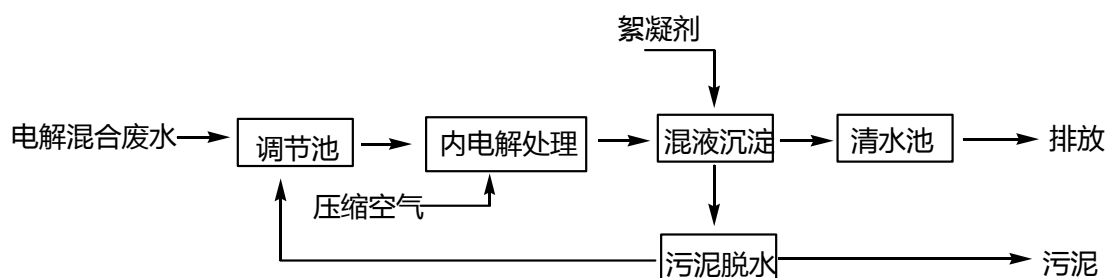
图 4.1-13 微电解法预处理混合废水
