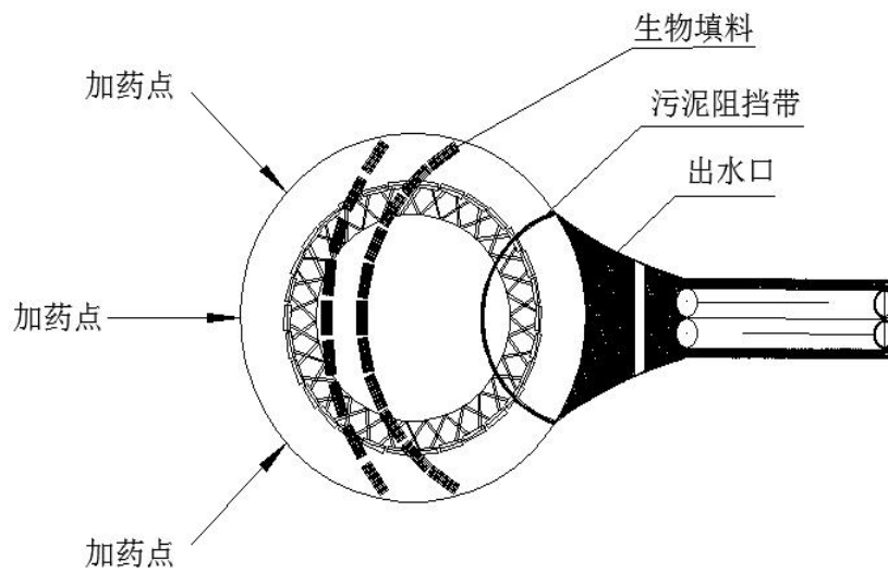
图 A.1 生物填料布置示意图 (圆形): 适用于圆形集水池
