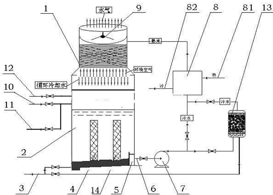
图 B.1 机械通风冷却塔池构造示意图
